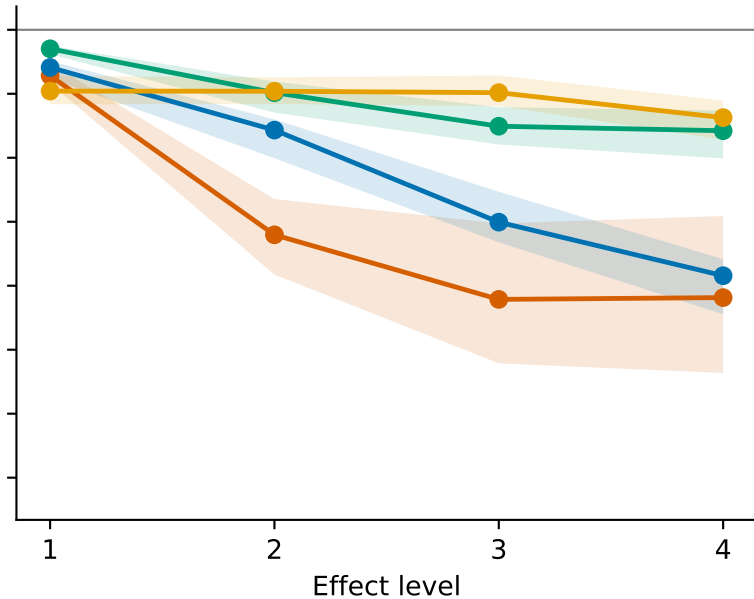
Spleeter (4-stem)
