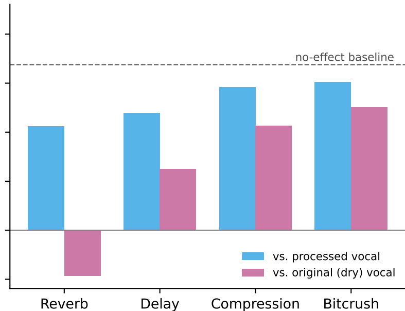
Spleeter (4-stem)
