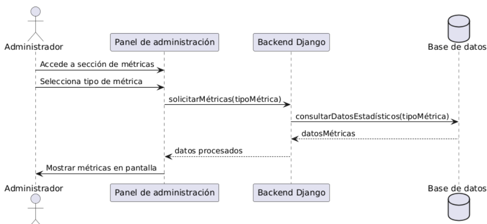
Figura 5.24: Diagrama de secuencia del caso de uso 19: Consultar métricas de uso
