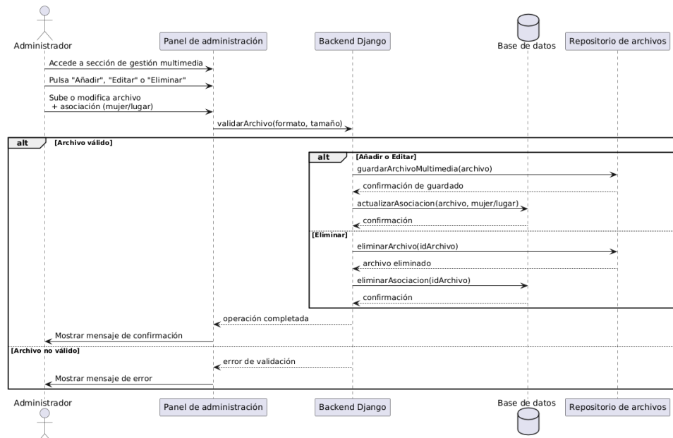
Figura 5.21: Diagrama de secuencia del caso de uso 18: Gestionar materiales multimedia
