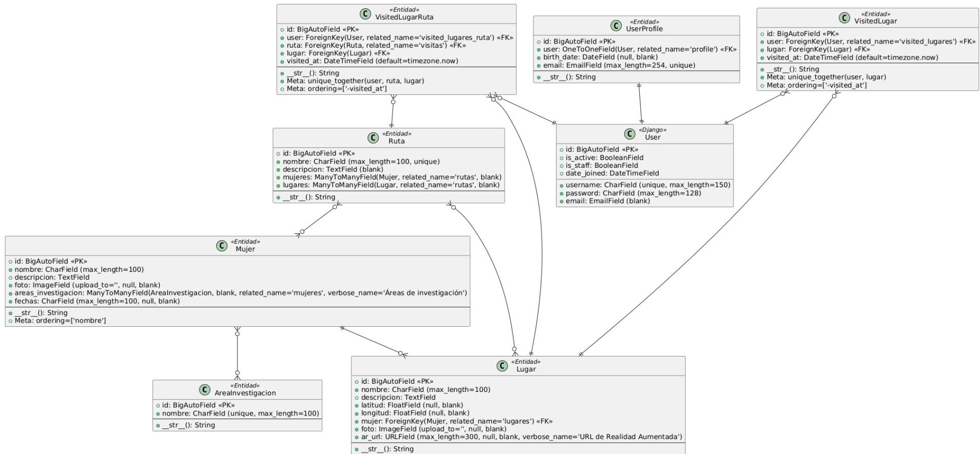
Figura 5.2: Diagrama de clases de la base de datos
