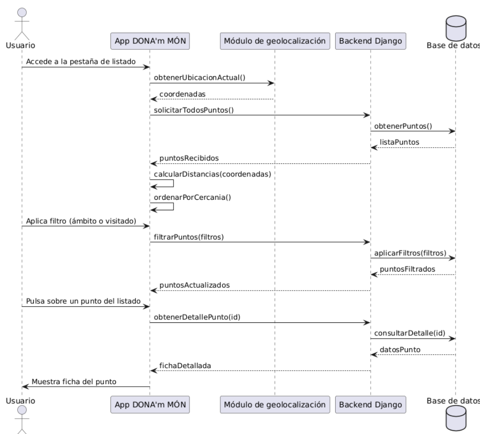
Figura 5.7: Diagrama de secuencia del caso de uso 4: Ver listado de puntos ordenado por cercanía
