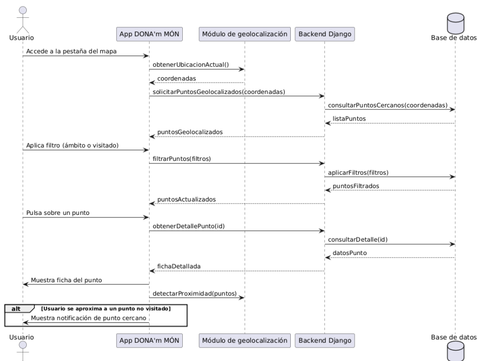
Figura 5.6: Diagrama de secuencia del caso de uso 3: Ver mapa con puntos de interés
