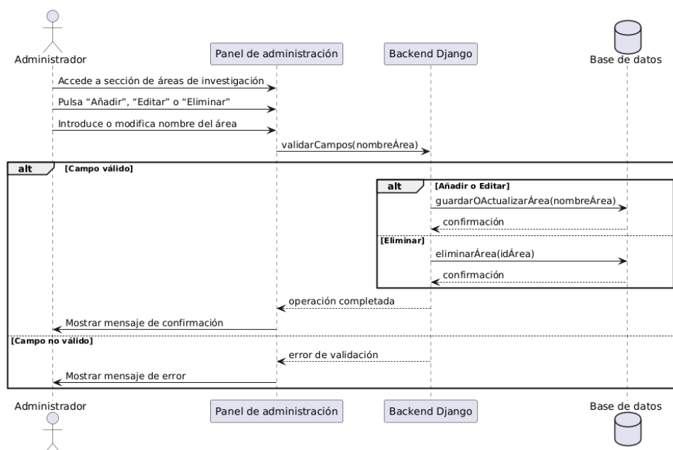
Figura 5.23: Diagrama de secuencia del caso de uso 20: Gestionar áreas de investigación
