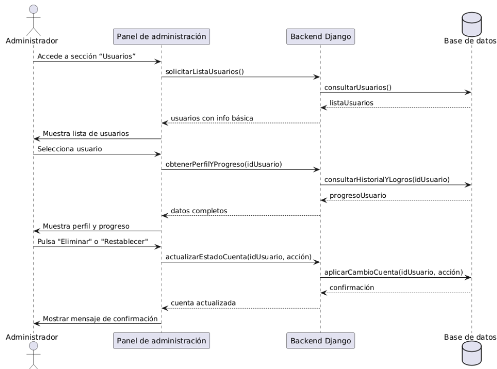
Figura 5.20: Diagrama de secuencia del caso de uso 17: Consultar lista de usuarios
