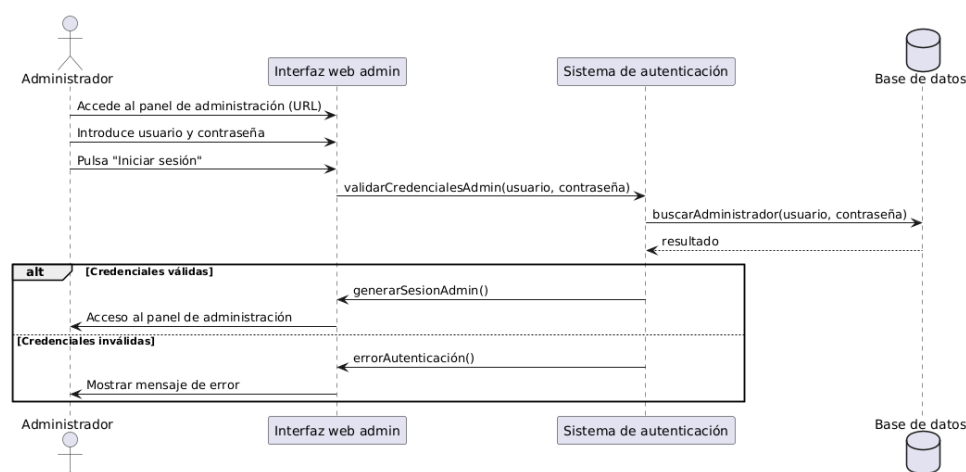
Figura 5.16: Diagrama de secuencia del caso de uso 13: Iniciar sesión como administrador
