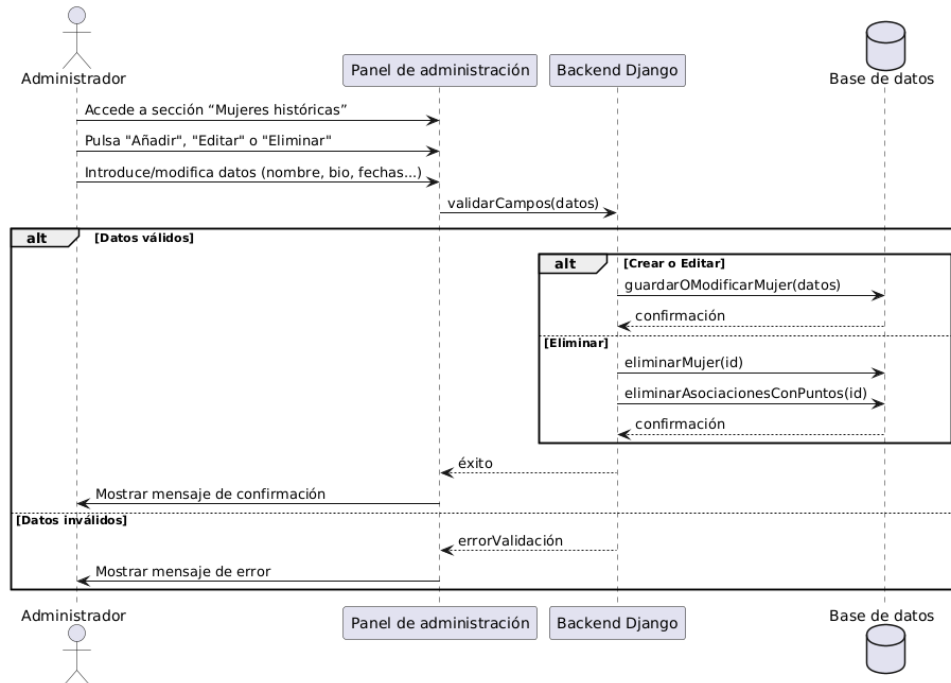
Figura 5.17: Diagrama de secuencia del caso de uso 14: Gestionar mujeres históricas
