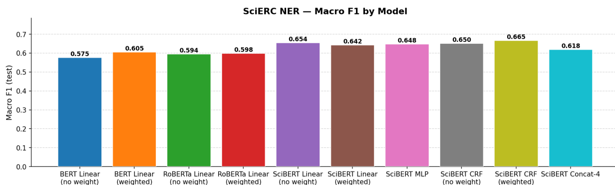
Рис. 5: Macro F1 по моделям (эксперимент 2)
