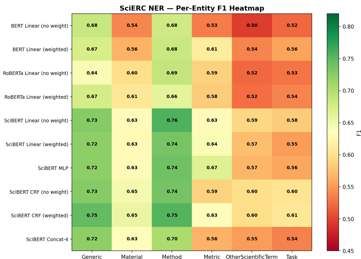
Рис. 6: Тепловая карта per-entity F1 (эксперимент 2)
