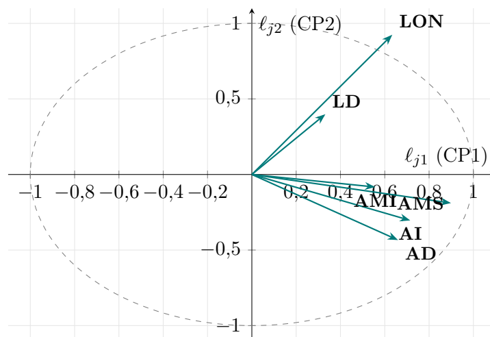
Figura 4: Cargas factoriales del problema P2: \ell_{ji} = v_{ji}\sqrt{\lambda_i} , no autovectores crudos.
