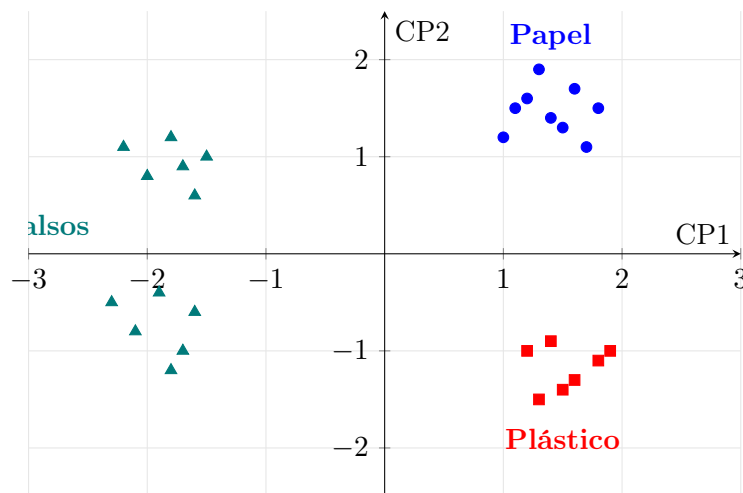
Figura 3: Reconstrucción de la dispersión de billetes en CP1-CP2 (P2).
