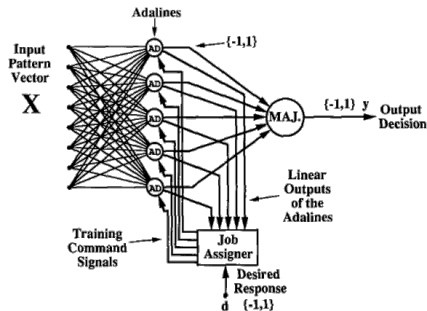
Fig. 15: Madaline I - Adalines signum + lógica fija .
