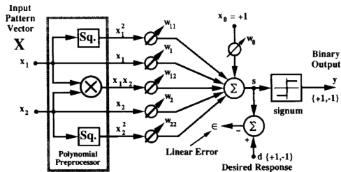
Fig. 6: Adaline con preprocesador polinomial fijo.
