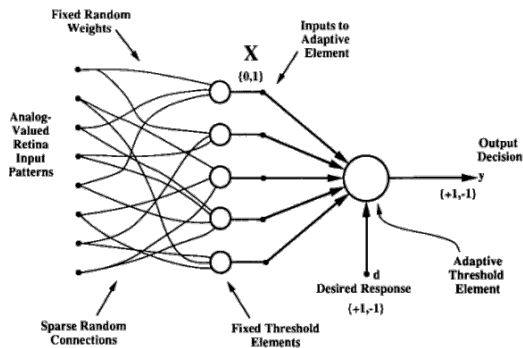
Fig. 13: el \alpha -Perceptrón de Rosenblatt - primera capa
