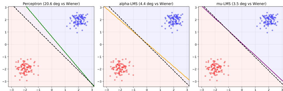
Fronteras aprendidas por cada regla vs. la solución de Wiener (datos separables).
