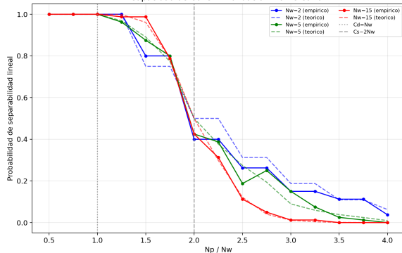
E1: Capacidad de Cover -- Validacion Monte Carlo
