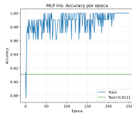
E6: MLP 4-8-3 en Iris (91.1 % test).
