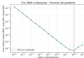
E7: error del gradiente y costo.
