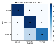
E6: MLP 4-8-3 en Iris (91.1 % test).
