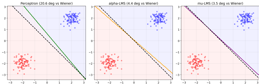
E2-E3: fronteras aprendidas vs. solución de Wiener (datos gaussianos 2D).
