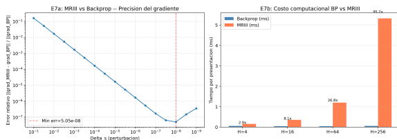
E7: error del gradiente y costo (red sigmoide).
