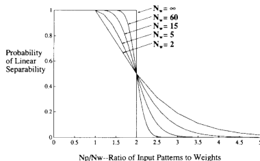
Fig. 5 del artículo (curvas teóricas de 1965).
