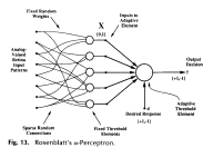
Fig. 13. Rosenblatt's \alpha -Perceptron.
