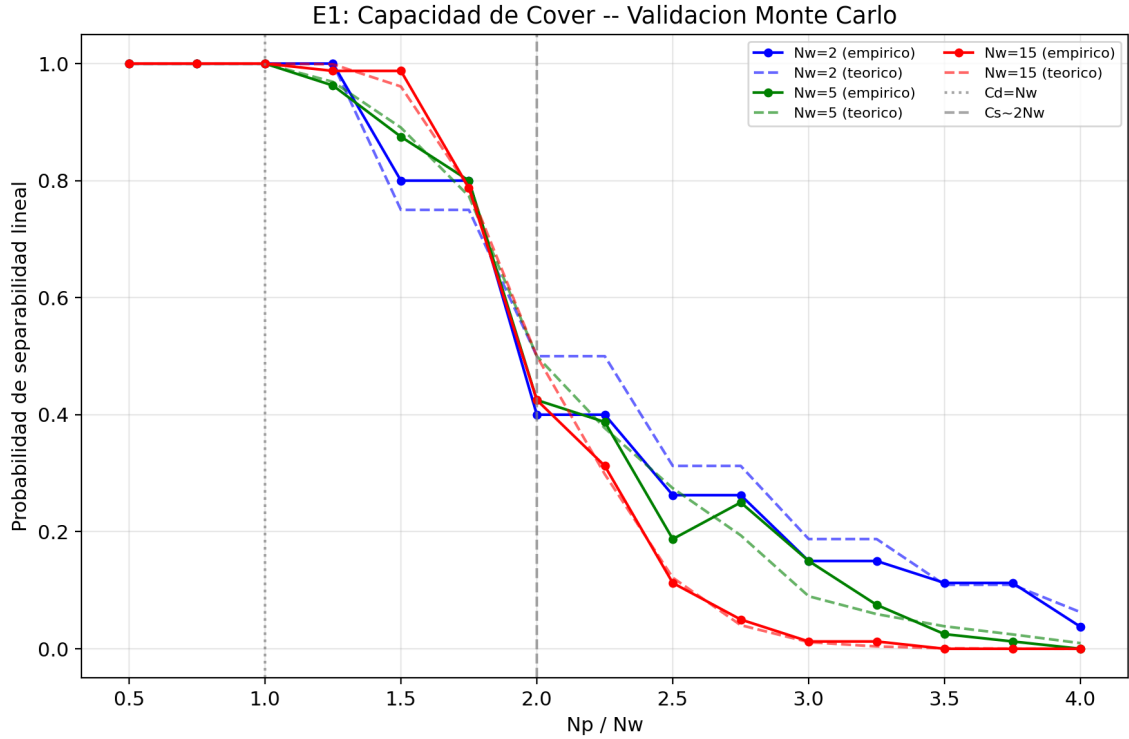
Figura 1: Probabilidad de separabilidad lineal: empírica (puntos) vs. fórmula teórica de Cover (curvas). Líneas verticales en C_d = N_w (punteada) y C_s \approx 2N_w (discontinua).
