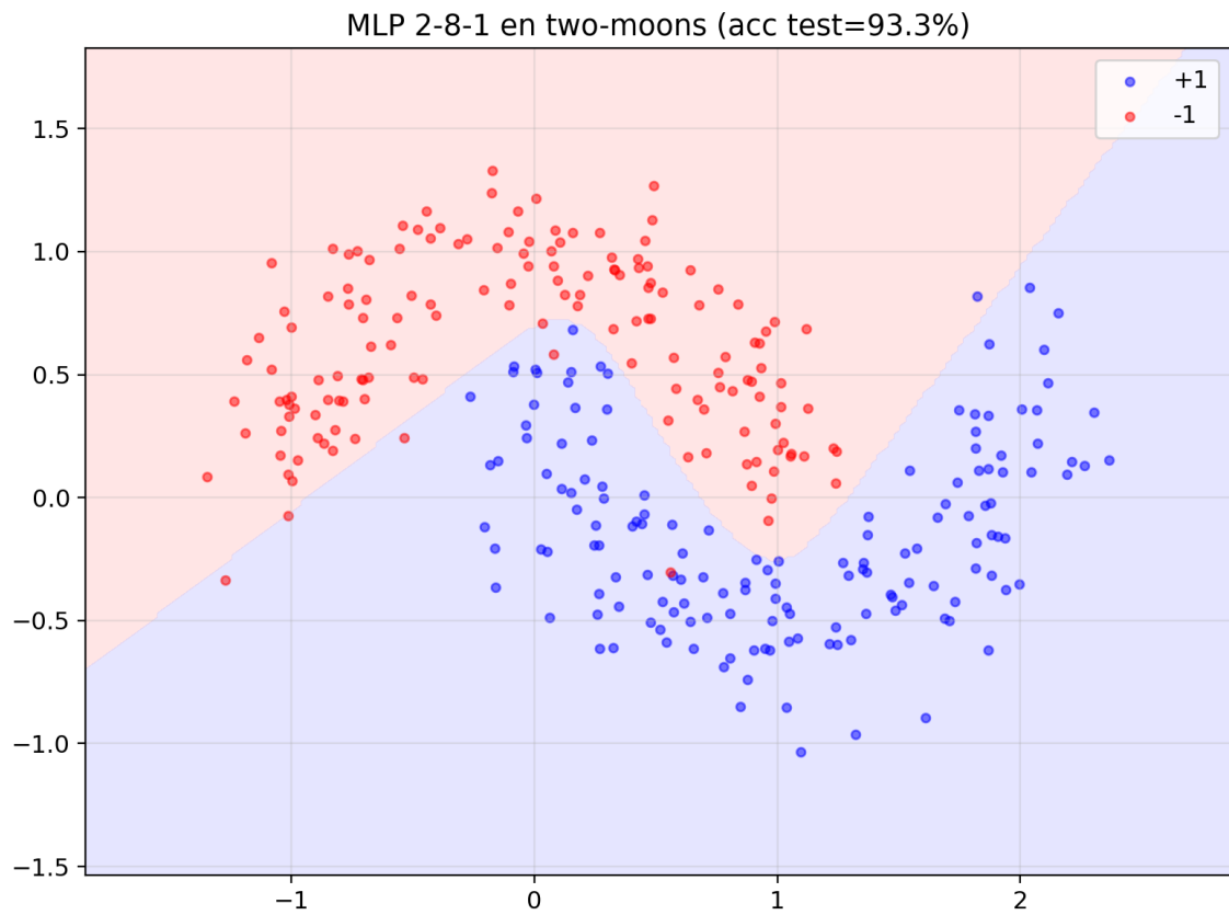
Figura 9: Regiones de decisión del MLP 2-8-1 en two-moons (93.3 % test).
