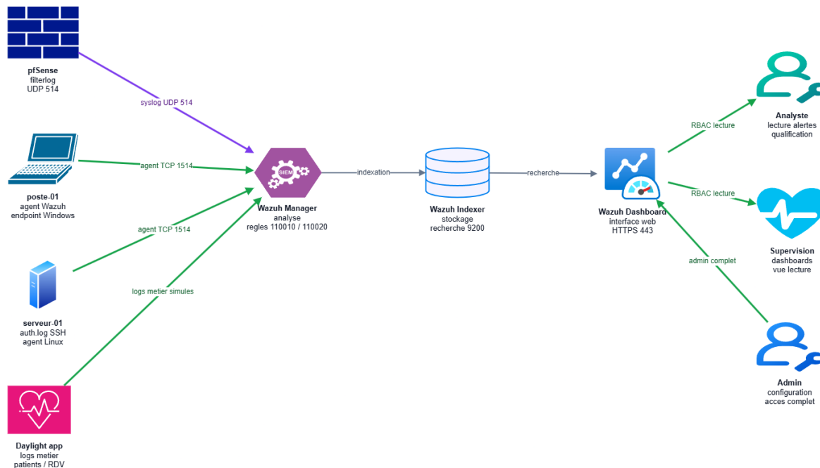
Figure compl?mentaire : cha?ne SOC Wazuh, depuis les sources de logs jusqu'aux r?les analyste, supervision et administrateur.
