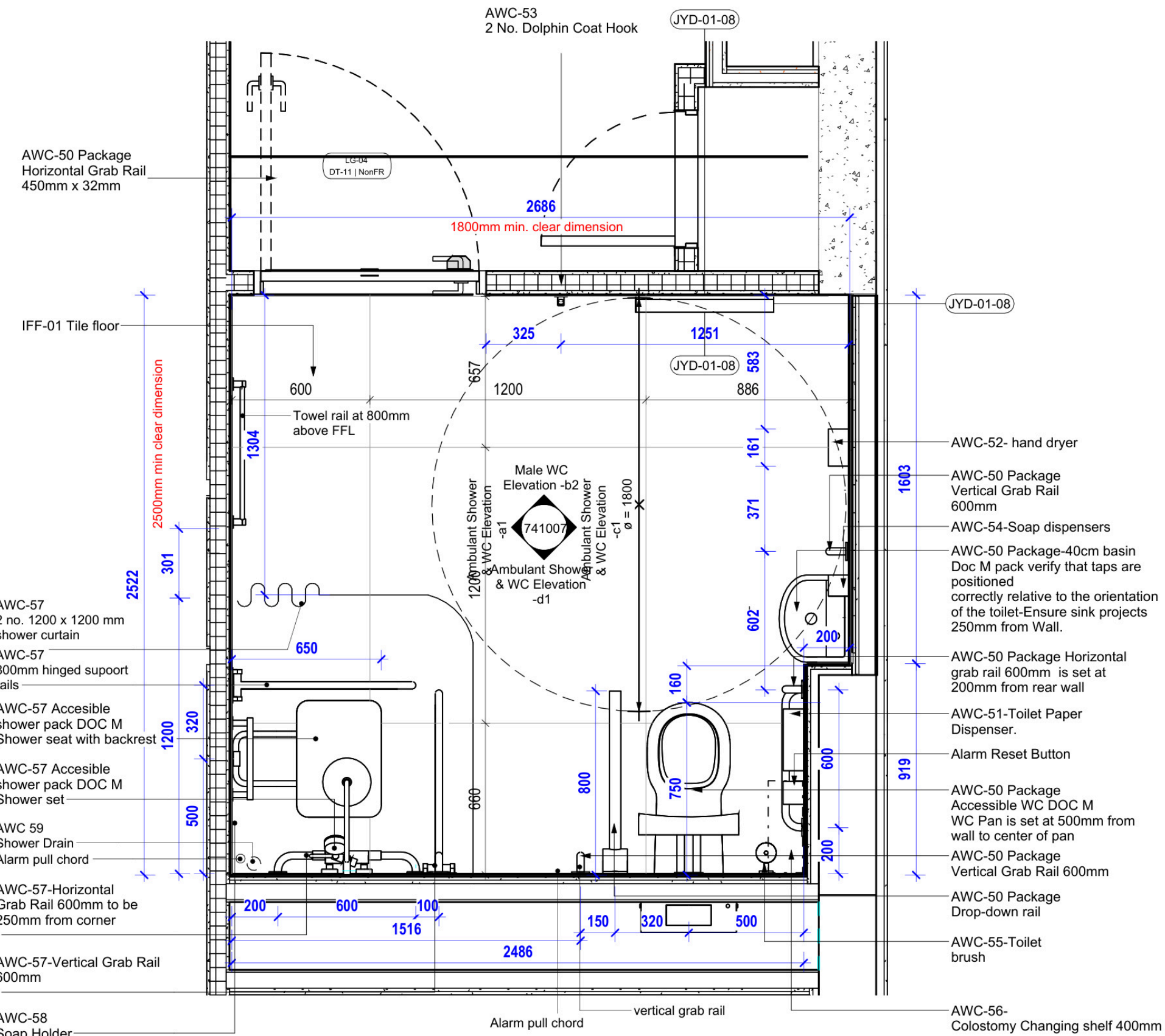
Ambulant Shower & WC Plan Basement -1 1 : 20
