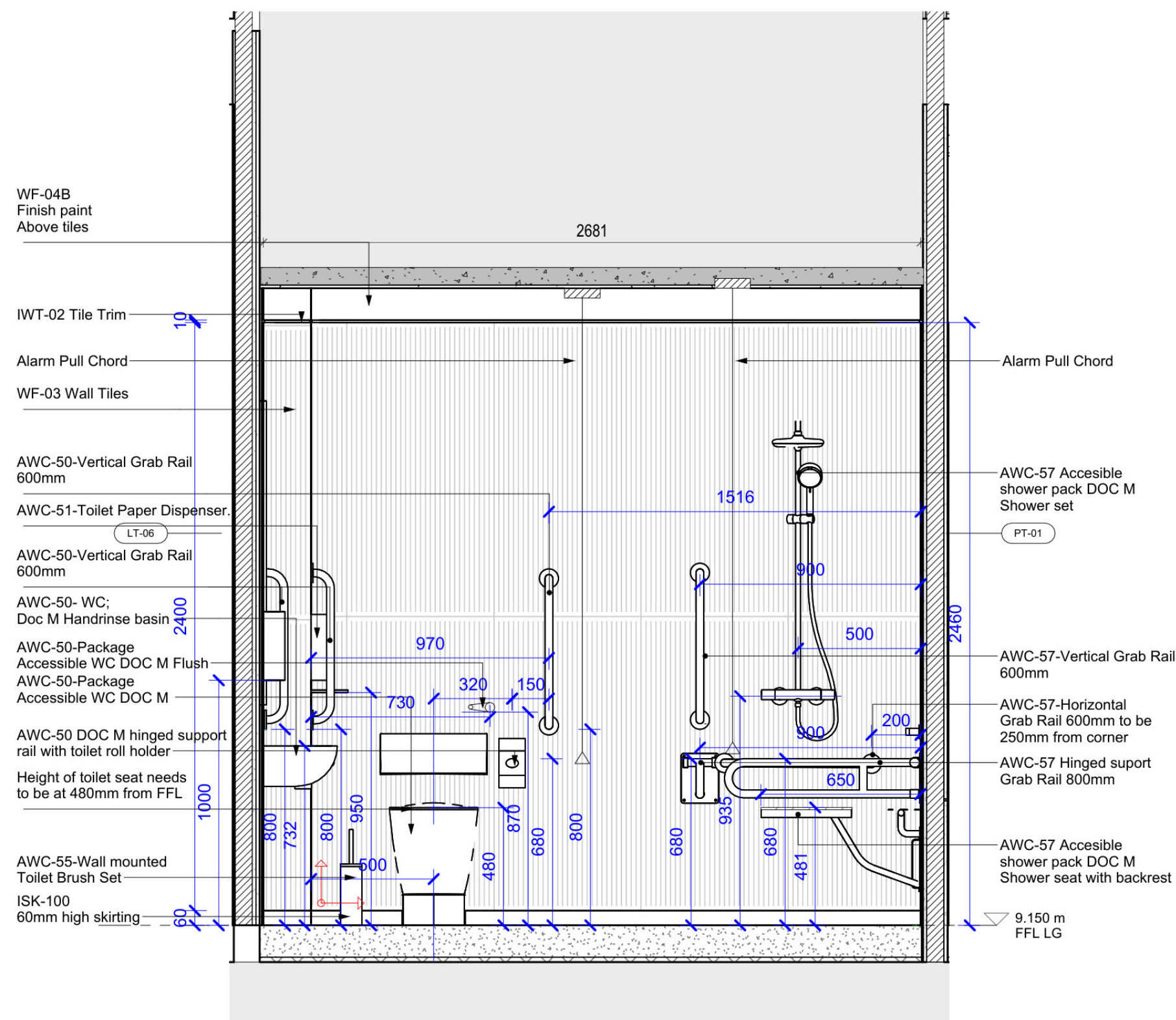
Ambulant Shower & WC Elevation -d1 1 : 20
