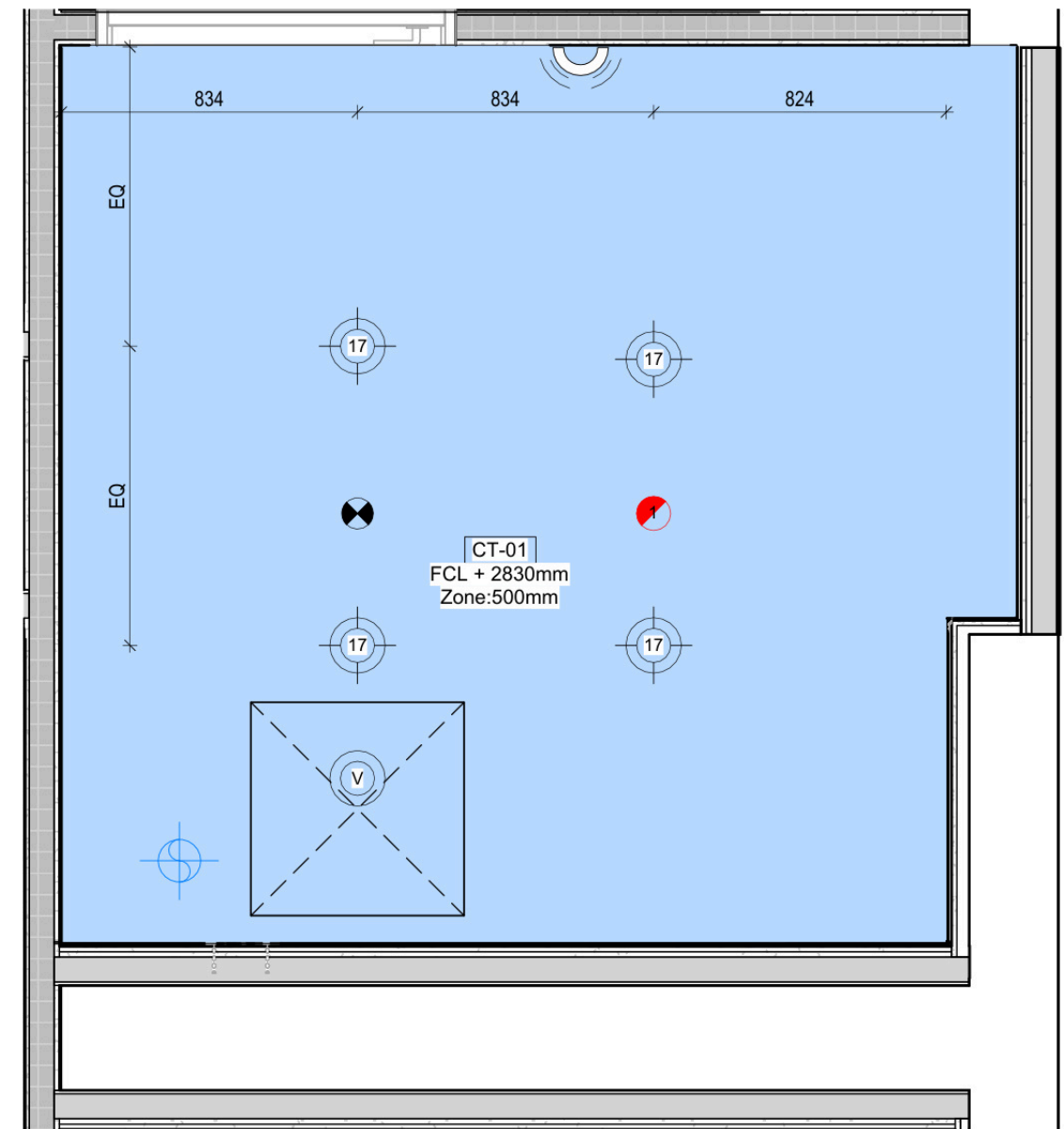
Ambulant Shower & WC B1 RCP 1 : 20
