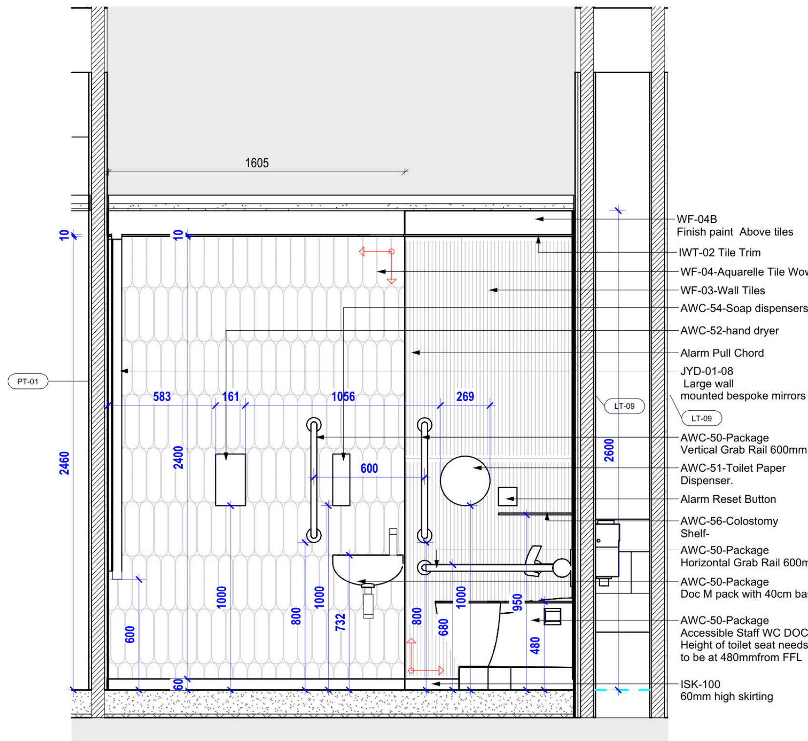
Ambulant Shower & WC Elevation -c1 1 : 20
