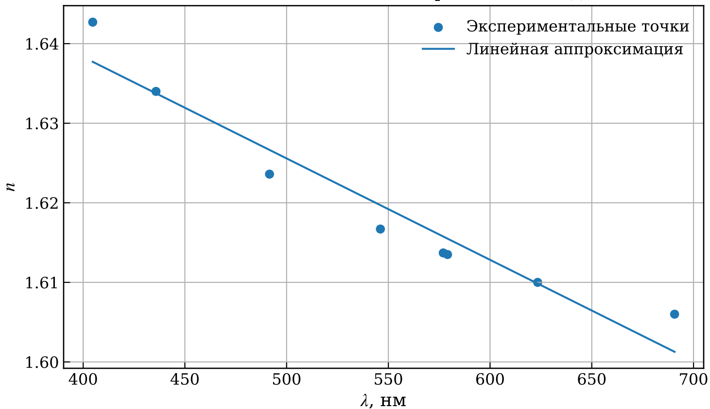
Зависимость показателя преломления n(\lambda)
