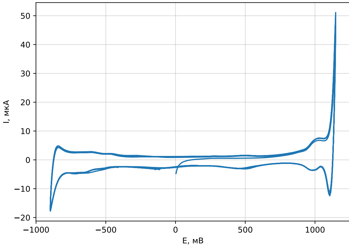
Циклическая ВАХ для Pt
