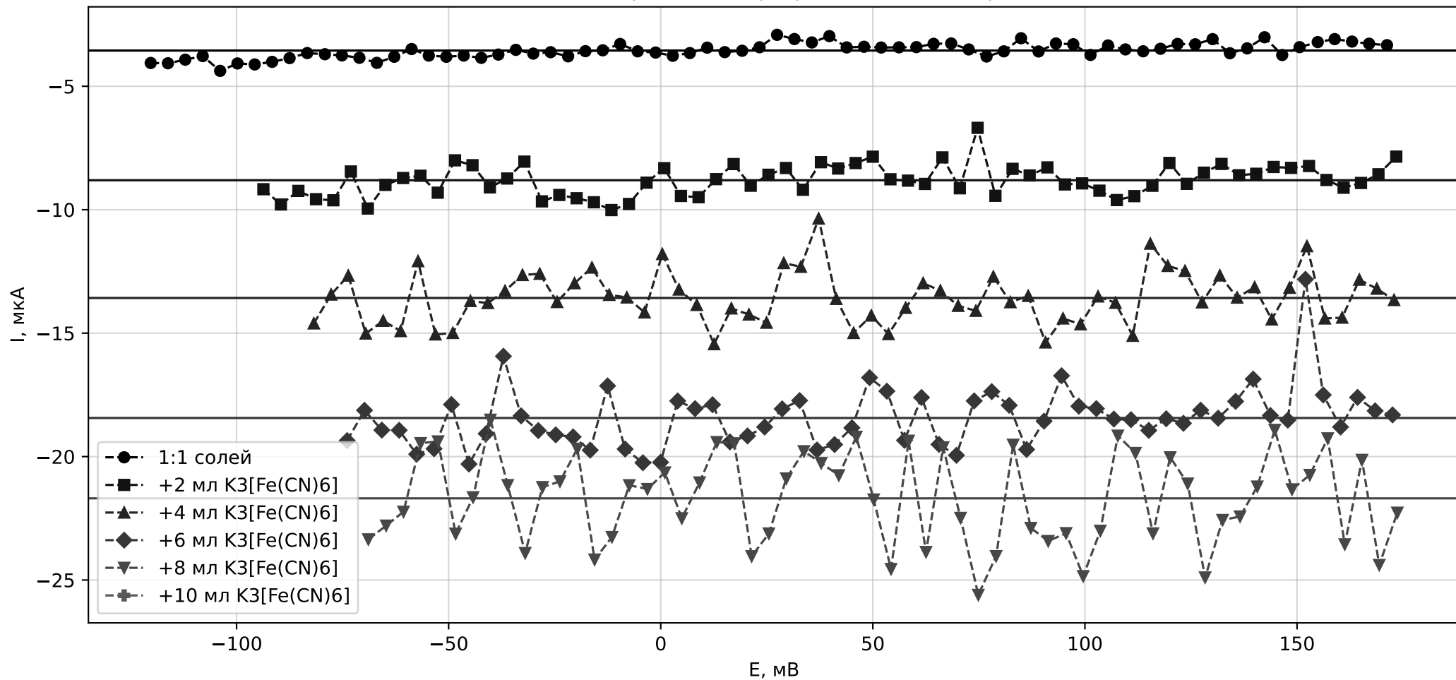
Зависимость тока от напряжения при разных концентрациях K_3[Fe(CN)_6]
