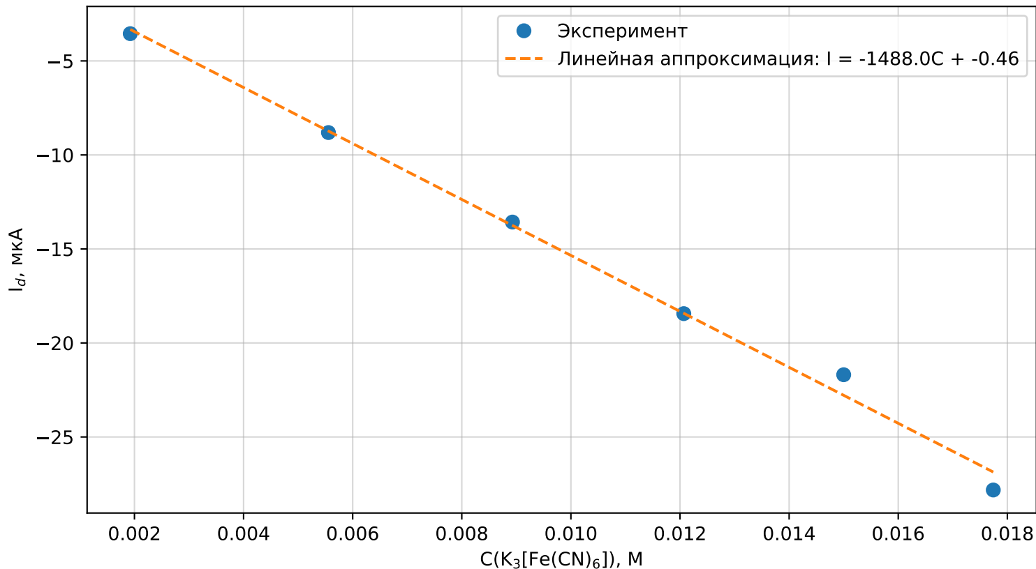
Зависимость предельного катодного диффузионного тока от концентрации K_3[Fe(CN)_6]
