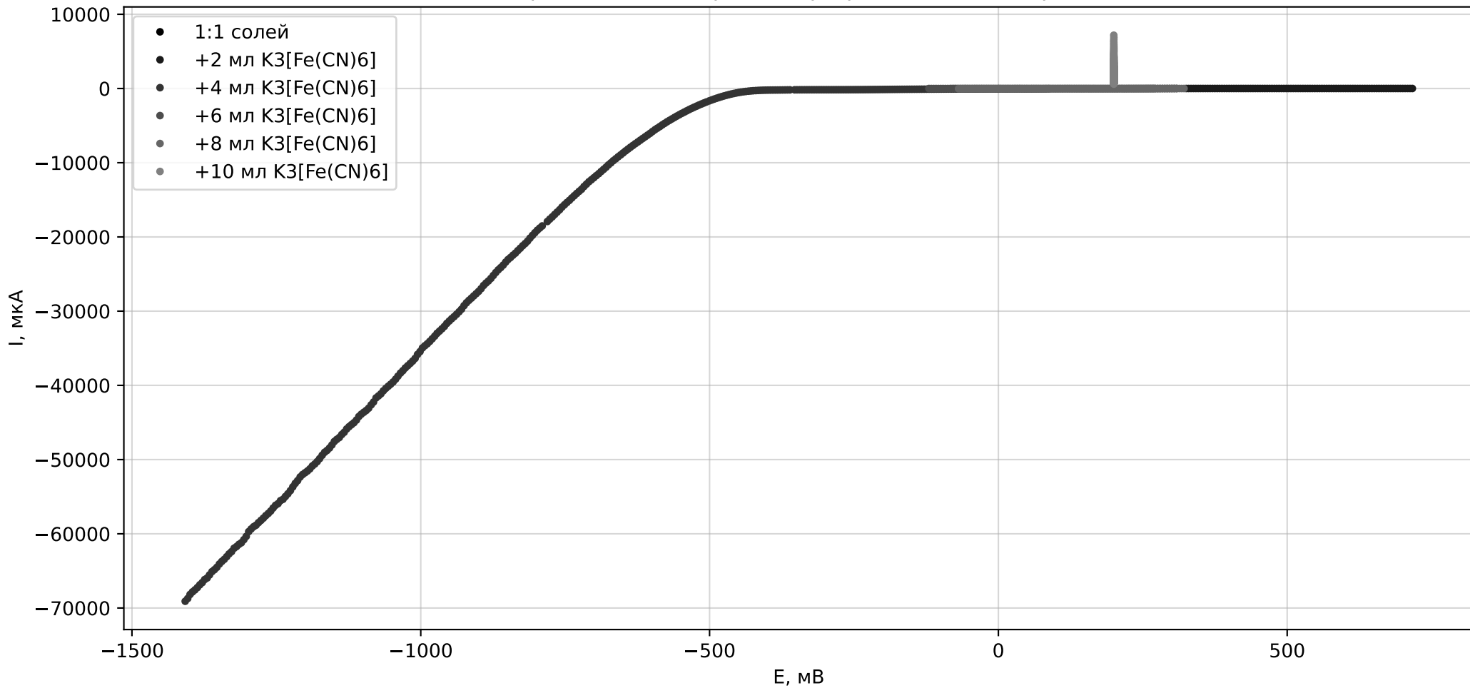
Поляризационные кривые при разных концентрациях
