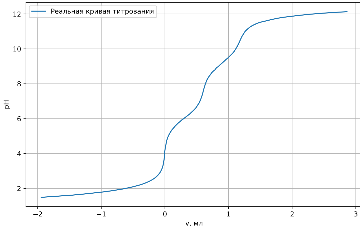
Экспериментальная кривая титрования
