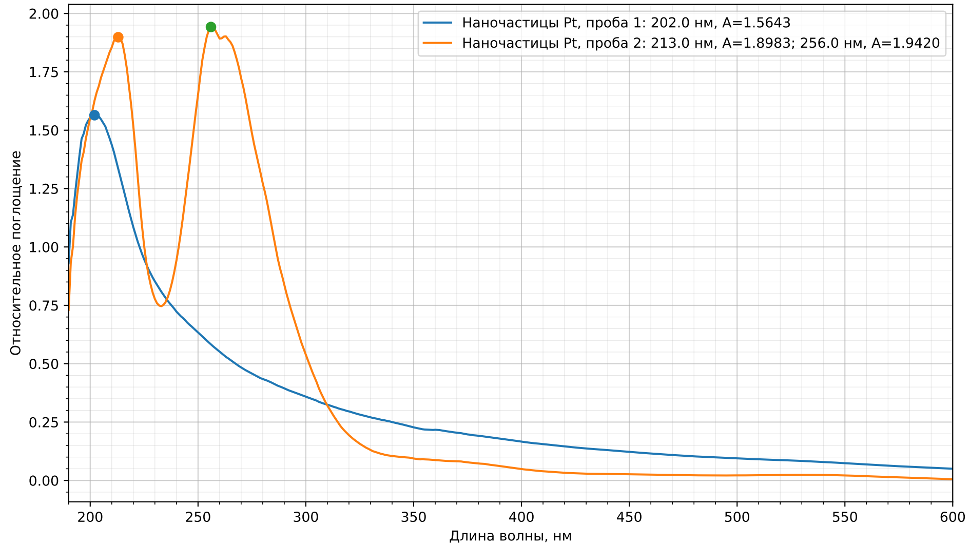
Спектры платины Pt
