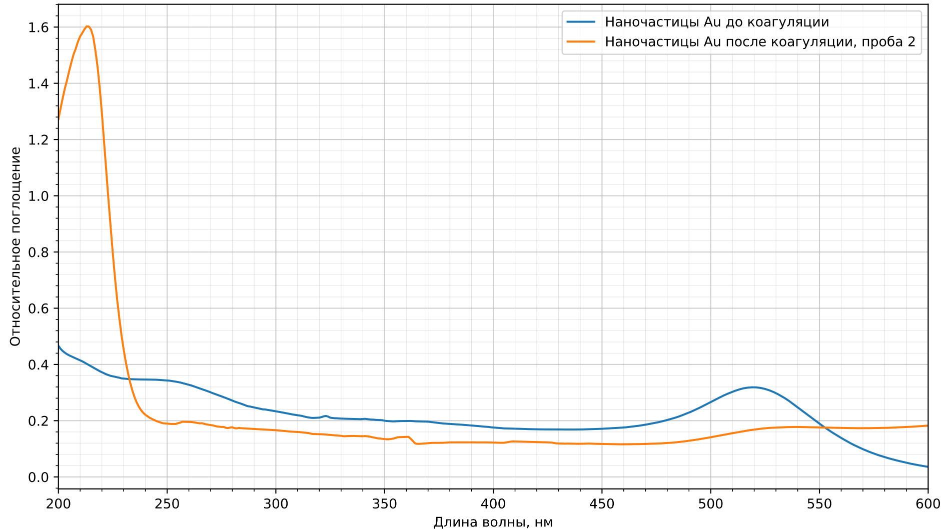
Спектры наночастиц Au до и после коагуляции
