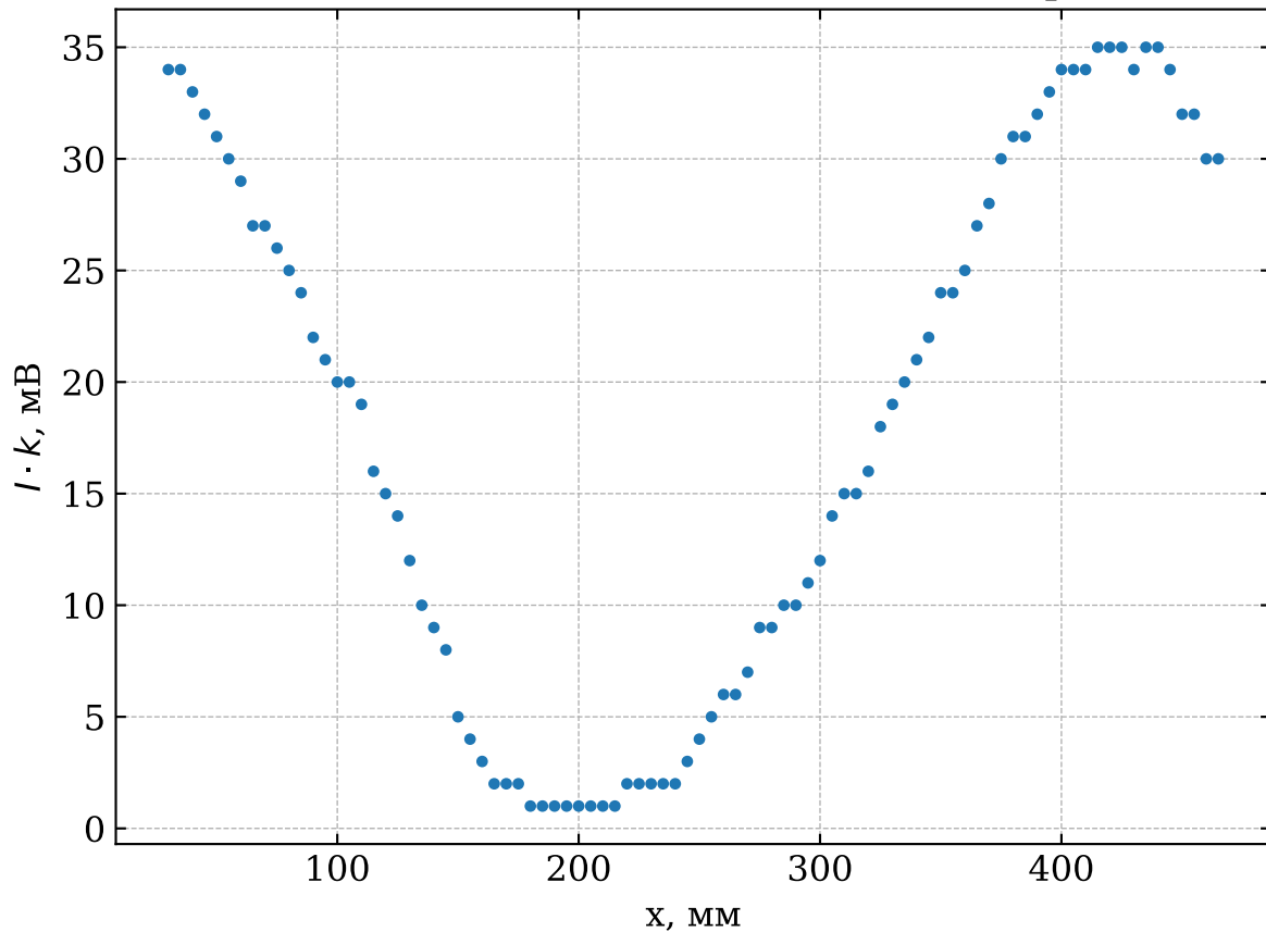
зависимость сигнала от смещения зеркала
