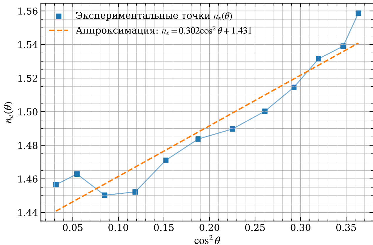
Зависимость n_e(\theta) от \cos^2 \theta
