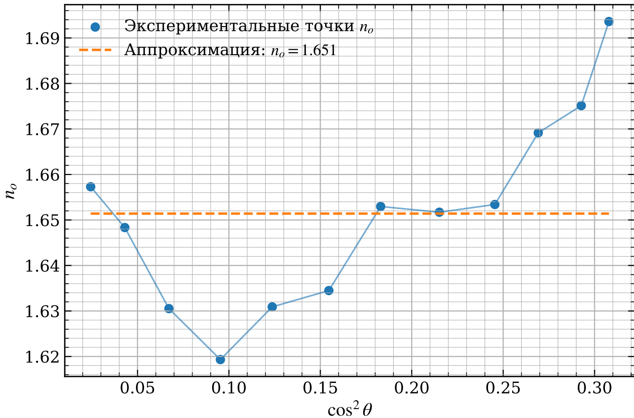
Зависимость n_o от \cos^2 \theta
