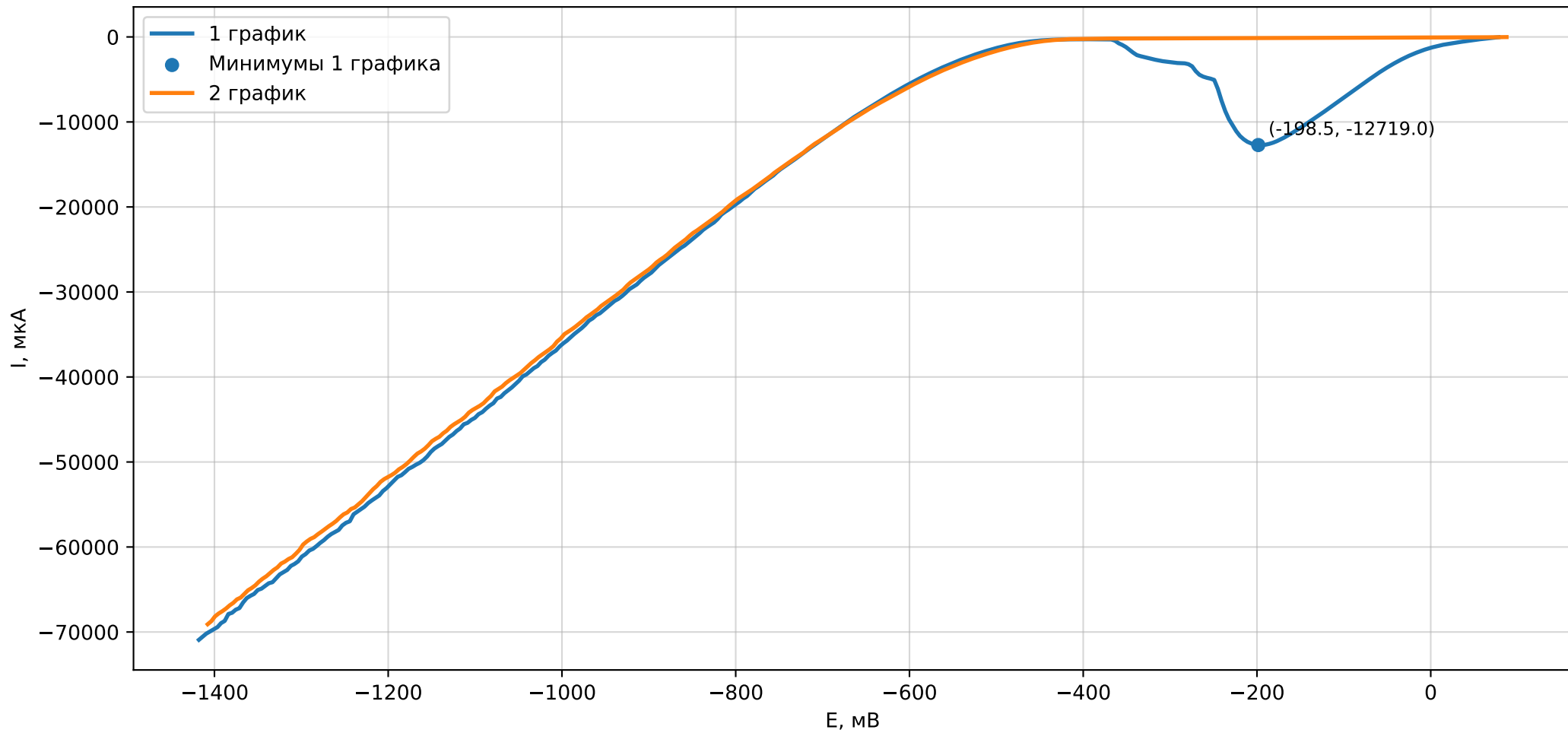
ВАХ катодной поляризации серебряной проволоки (очистка)
