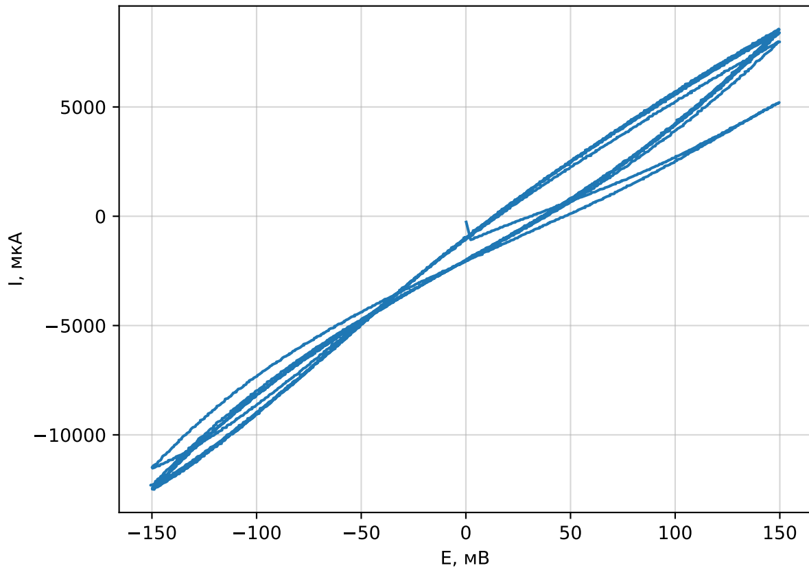
Циклическая ВАХ для AgCl
