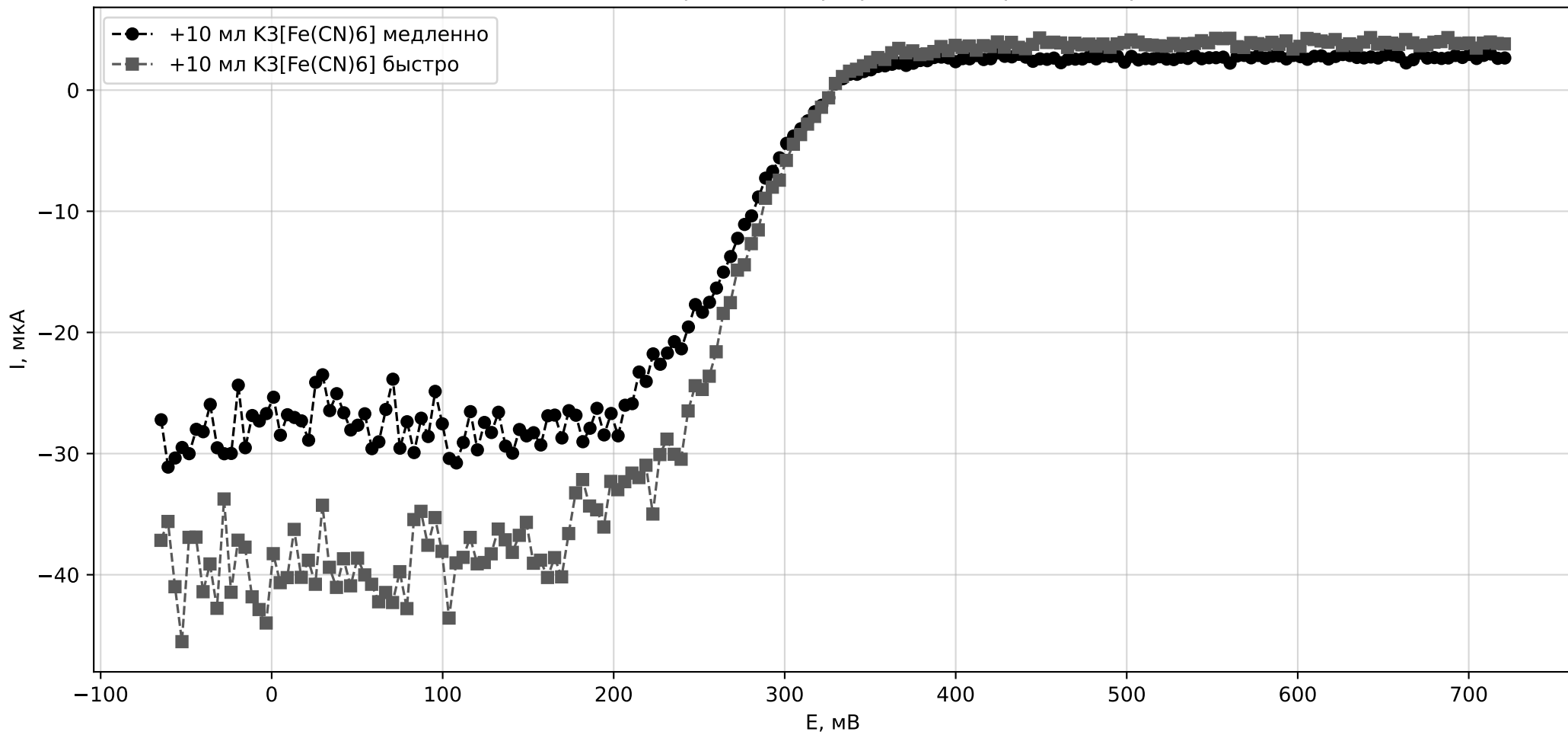
Зависимость тока от напряжения при разных скоростях перемешивания
