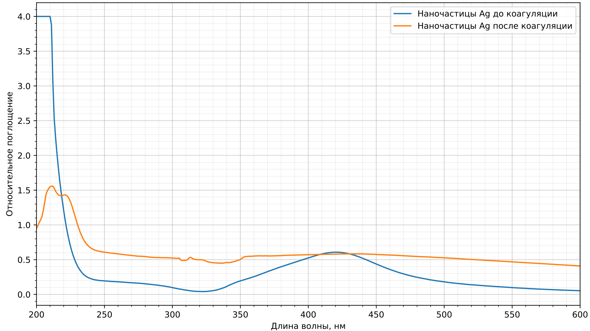
Спектры наночастиц Ag до и после коагуляции
