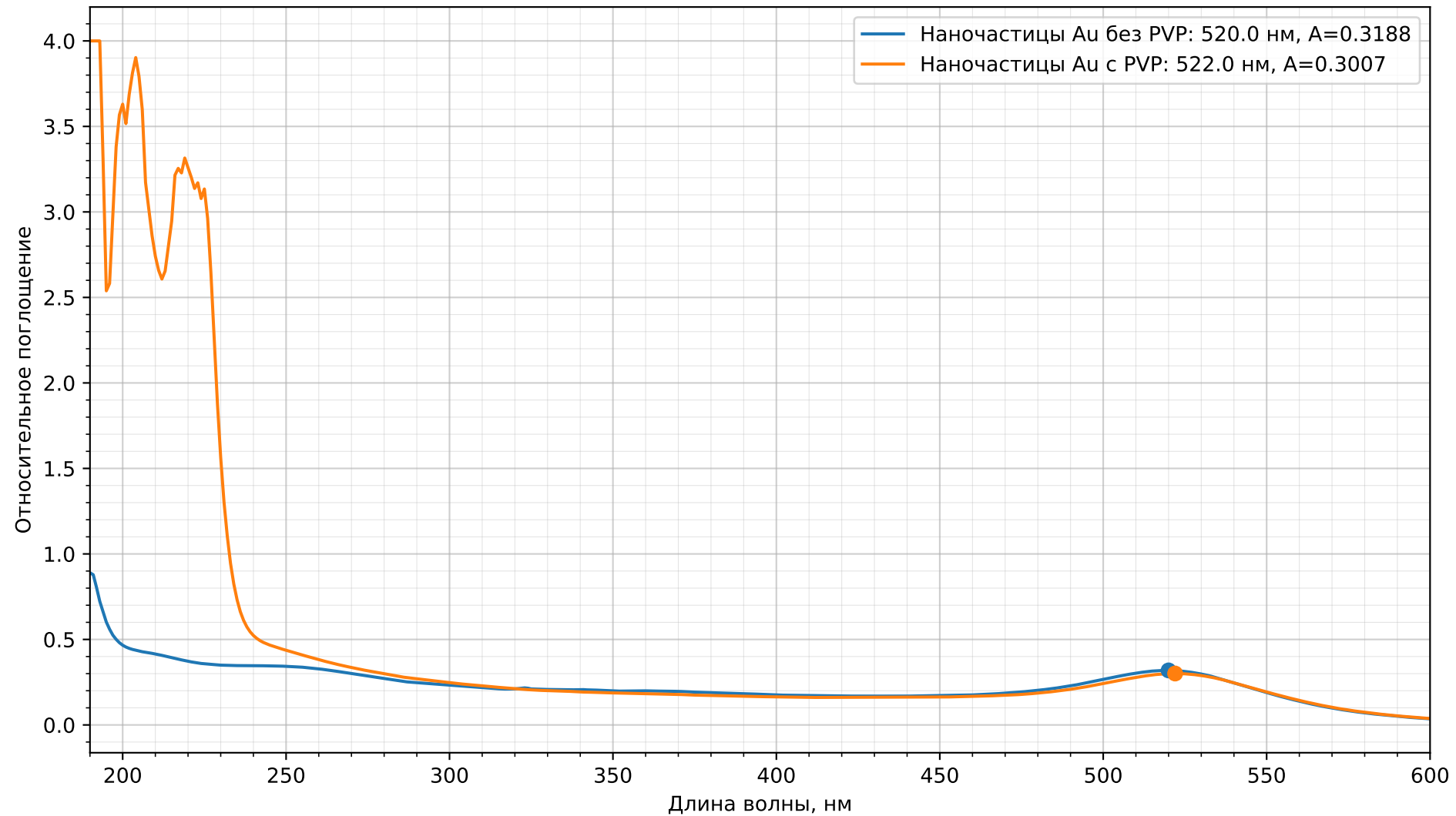
Спектры наночастиц Au с PVP и без PVP
