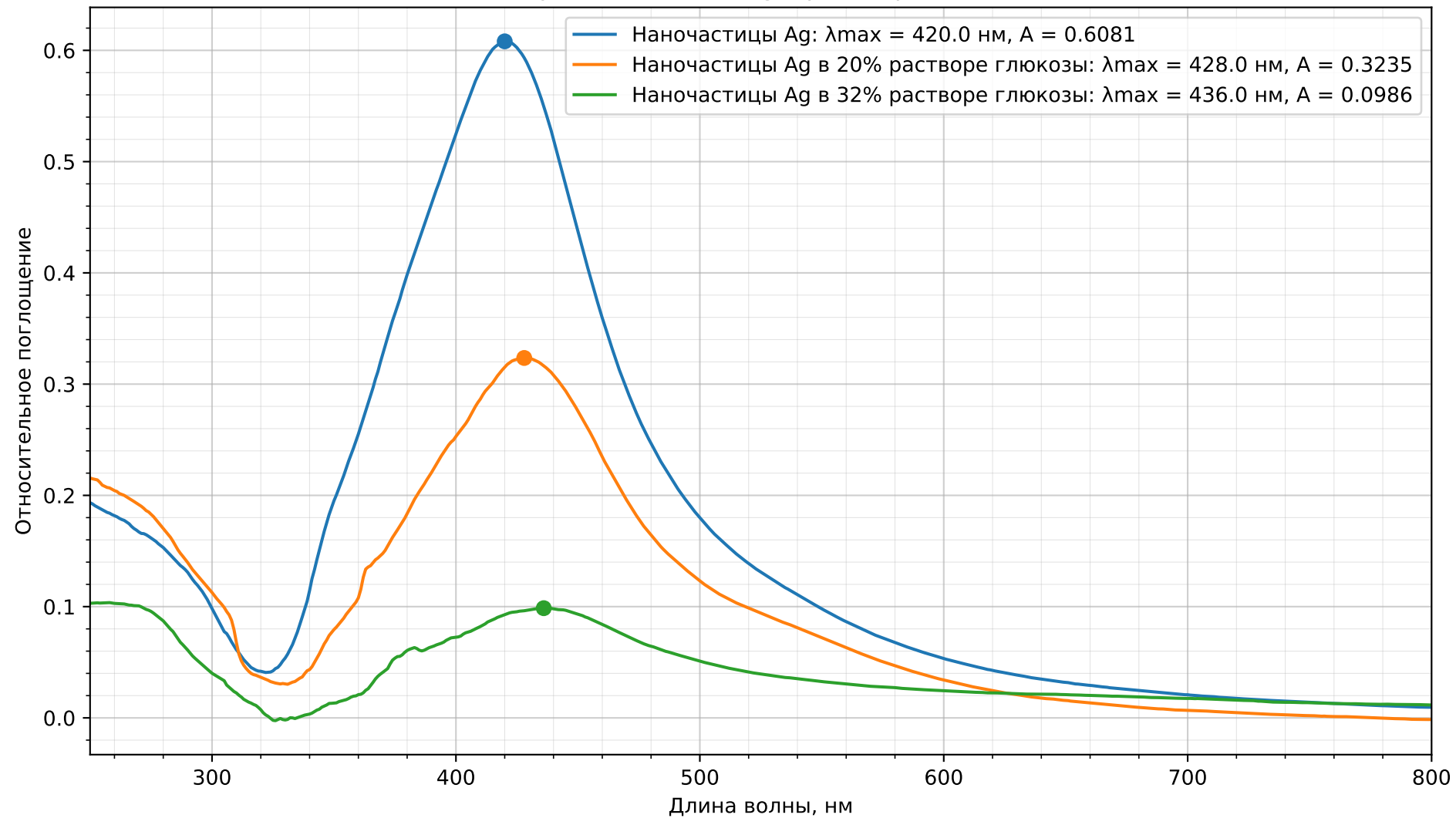
Спектры наночастиц Ag в растворах глюкозы
