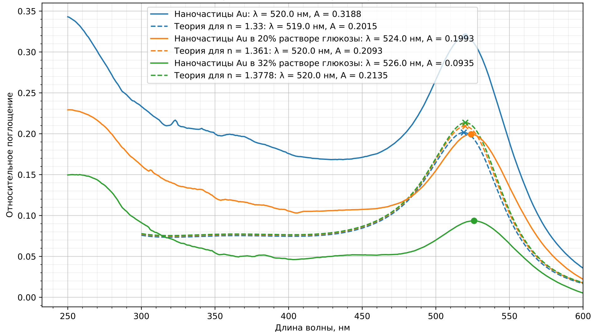
Спектры наночастиц Au в растворах глюкозы
