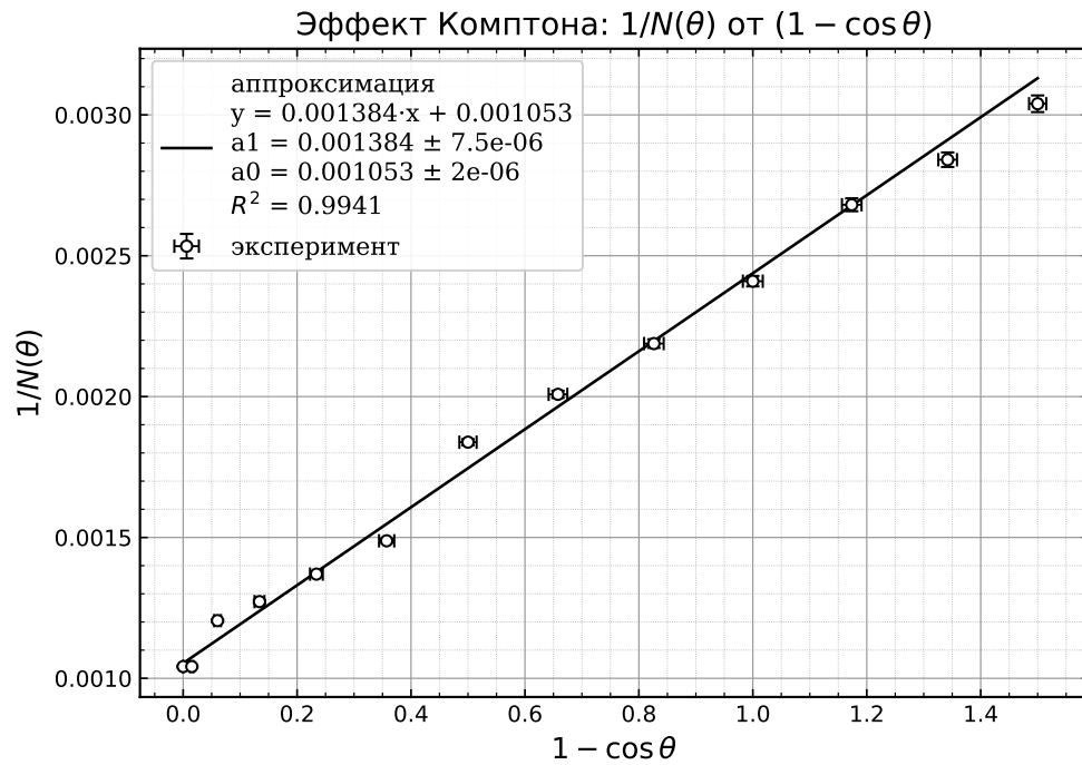
Рис. 1: Эффект Комптона на графите: 1/N(\theta) от (1 - \cos \theta) ; ^{137}\text{Cs} , E_\gamma = 661.657 кэВ.
