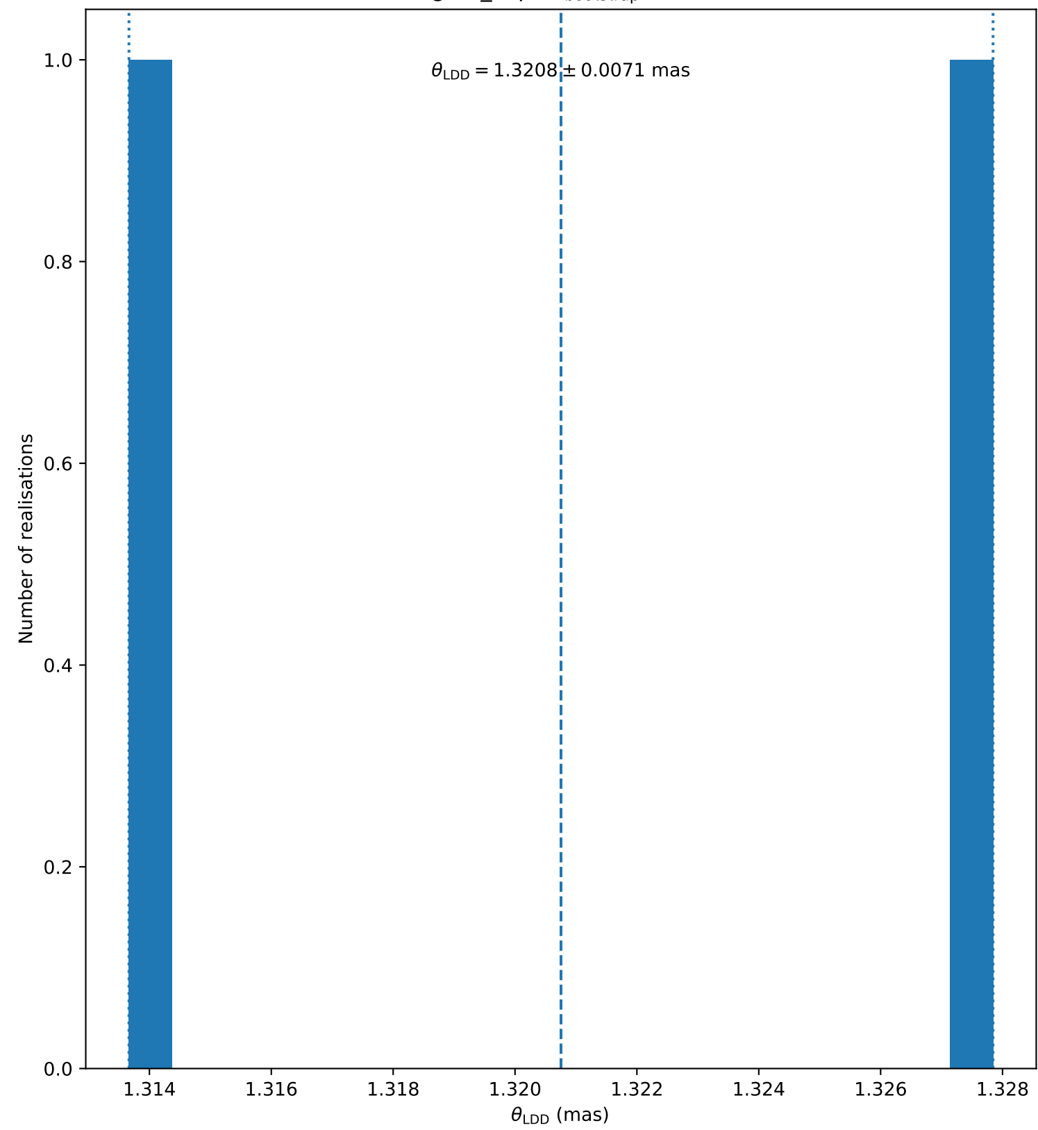
gam_Lep ( N_{\text{bootstrap}} = 2 )
