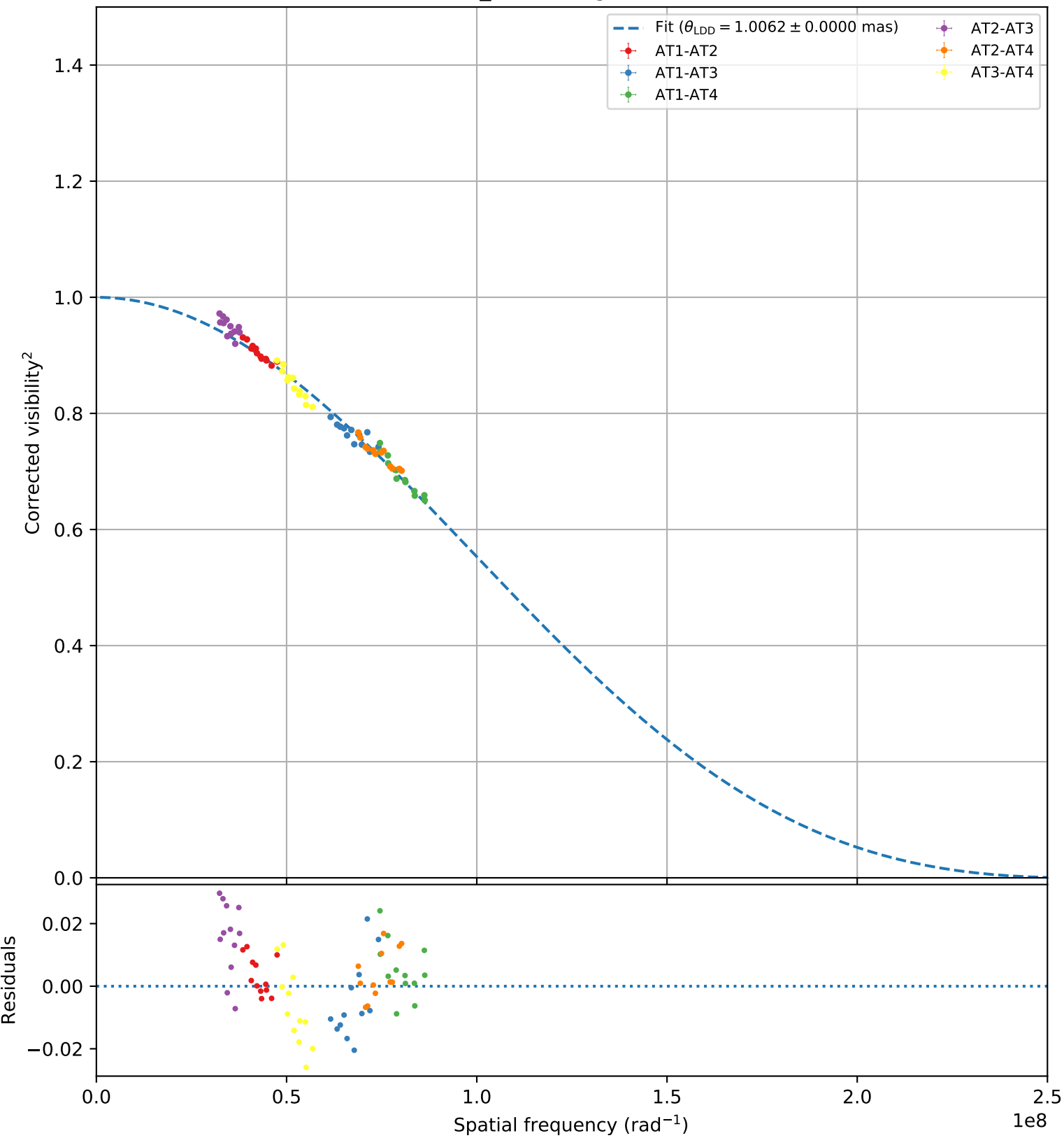
HR_2998 (bright, 104)
