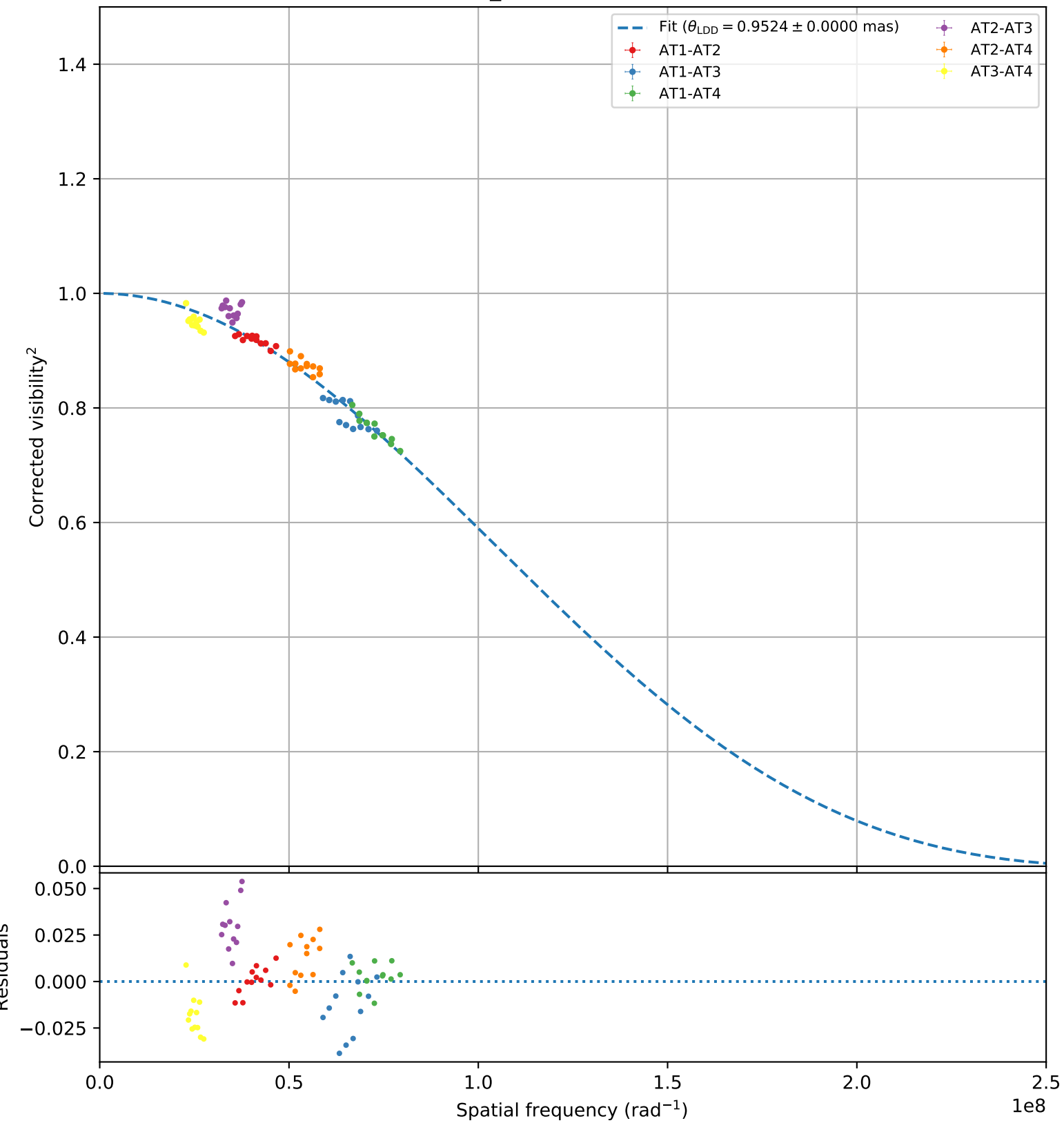
HR_2998 (faint, 104)
