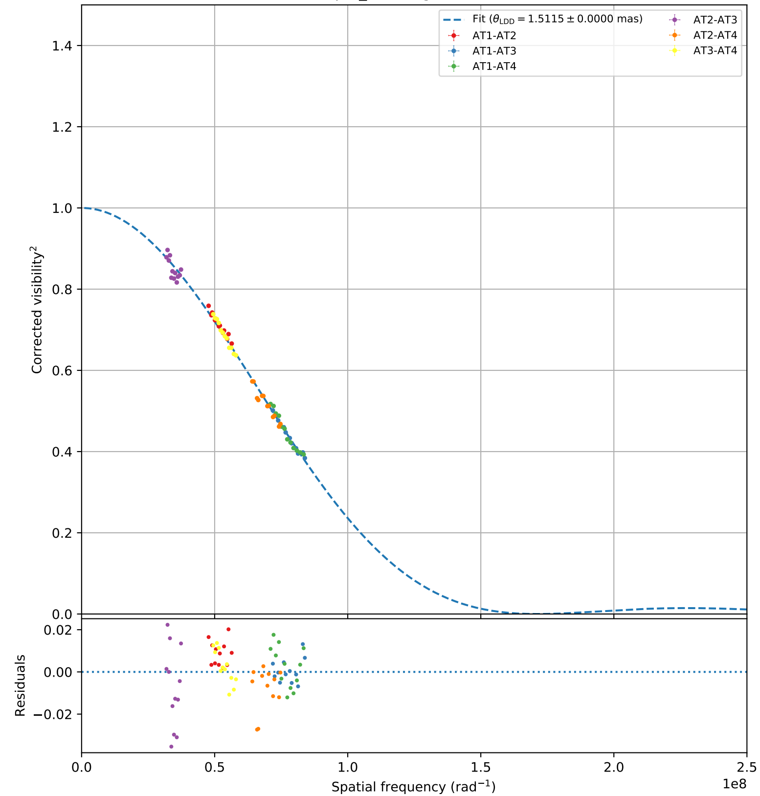
pi3_Ori (bright, 104)
