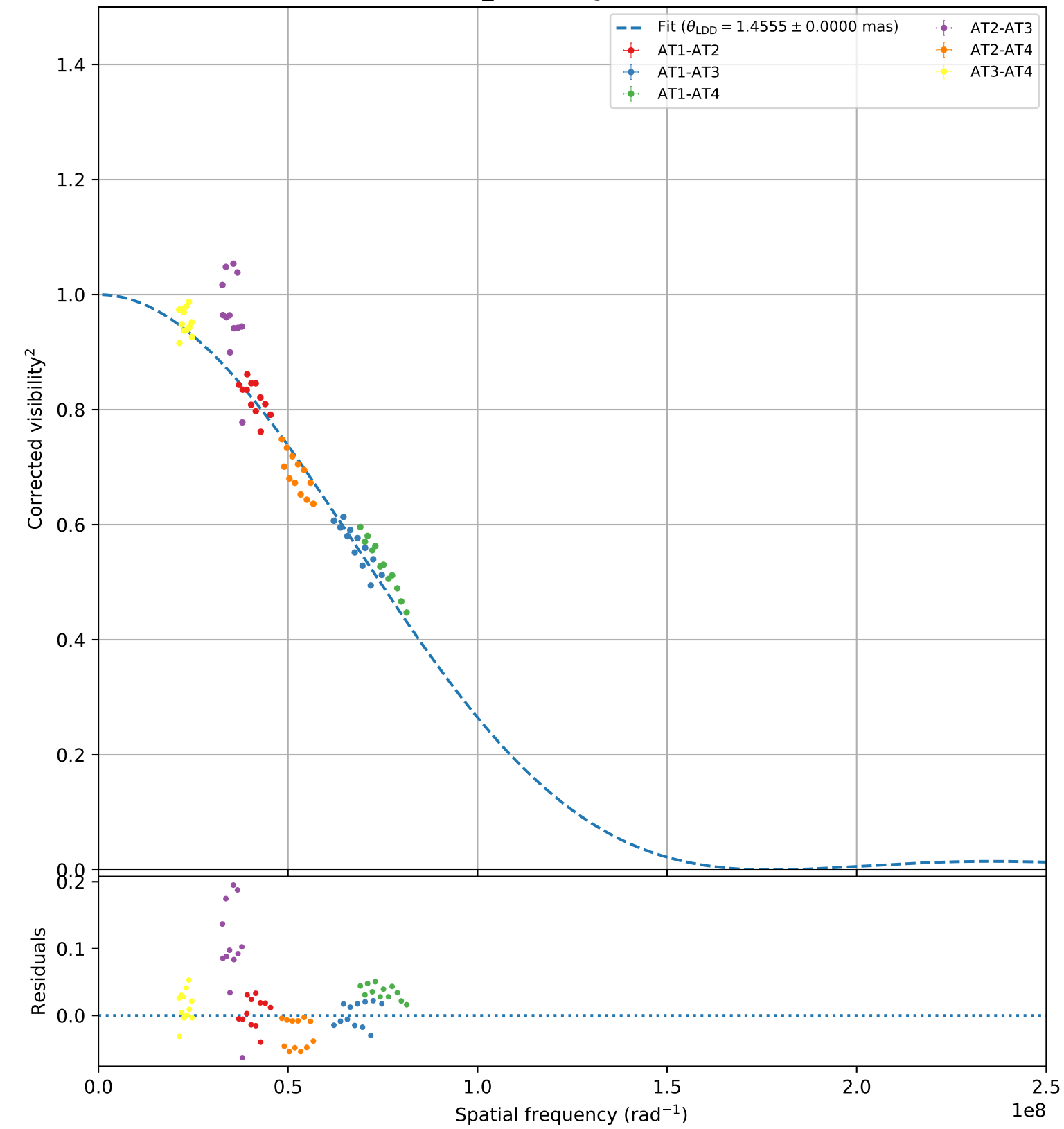
ksi_Gem (bright, 106)
