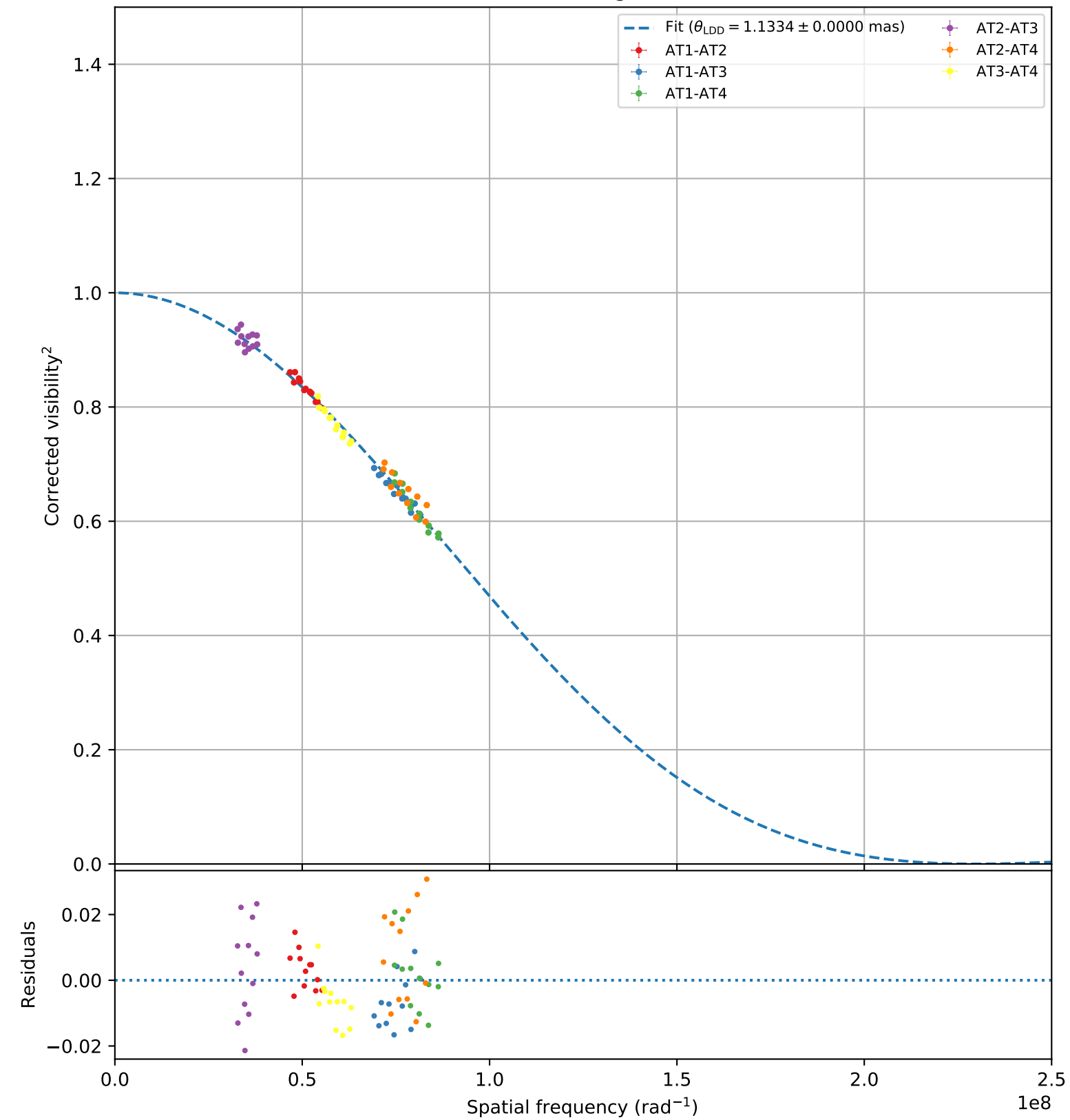
HD124850 (bright, 105)
