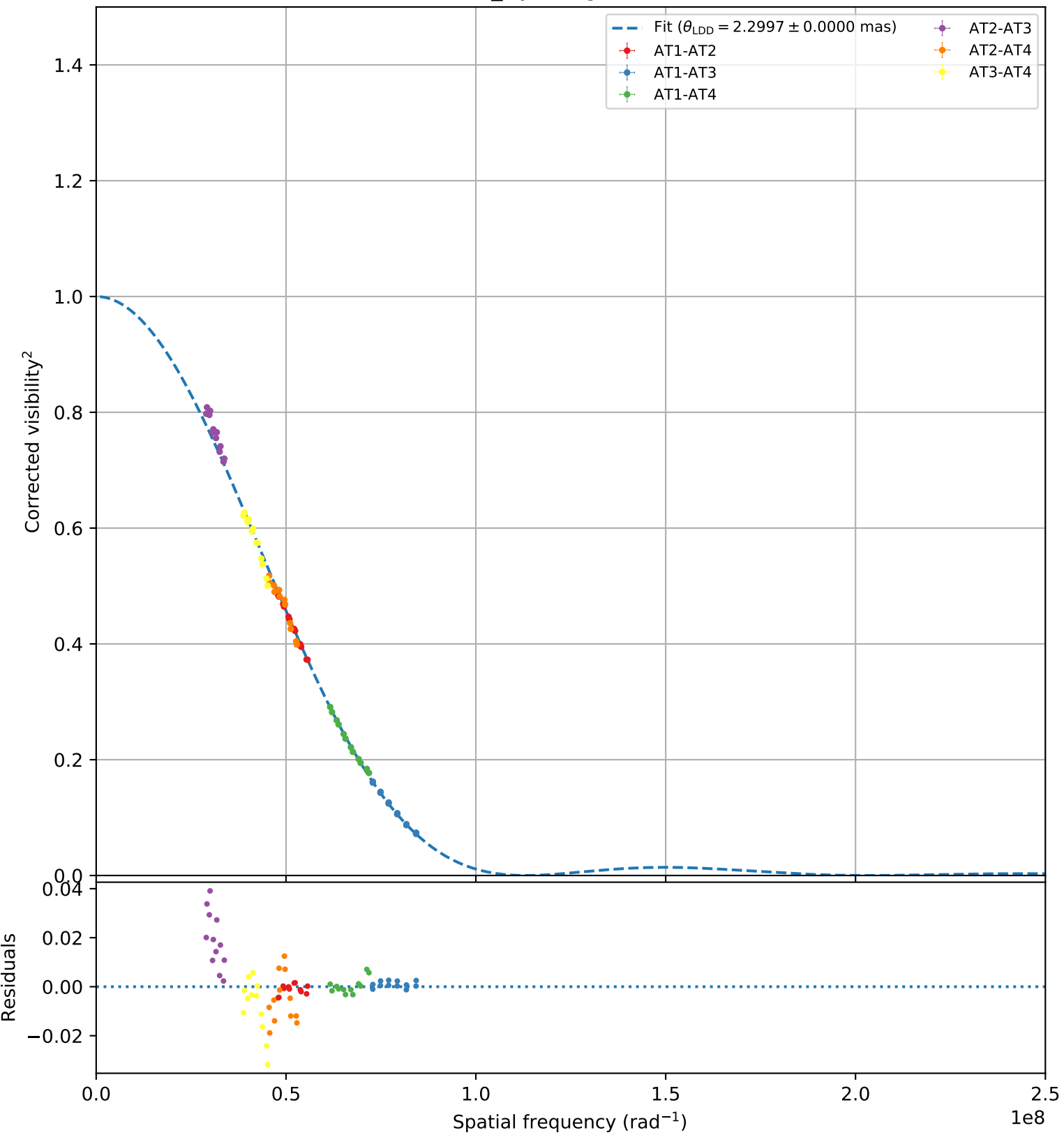
bet_Hyi (bright, 106)
