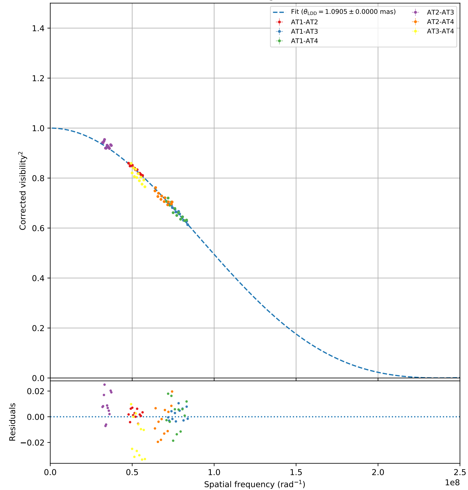
HD141004 (bright, 105)
