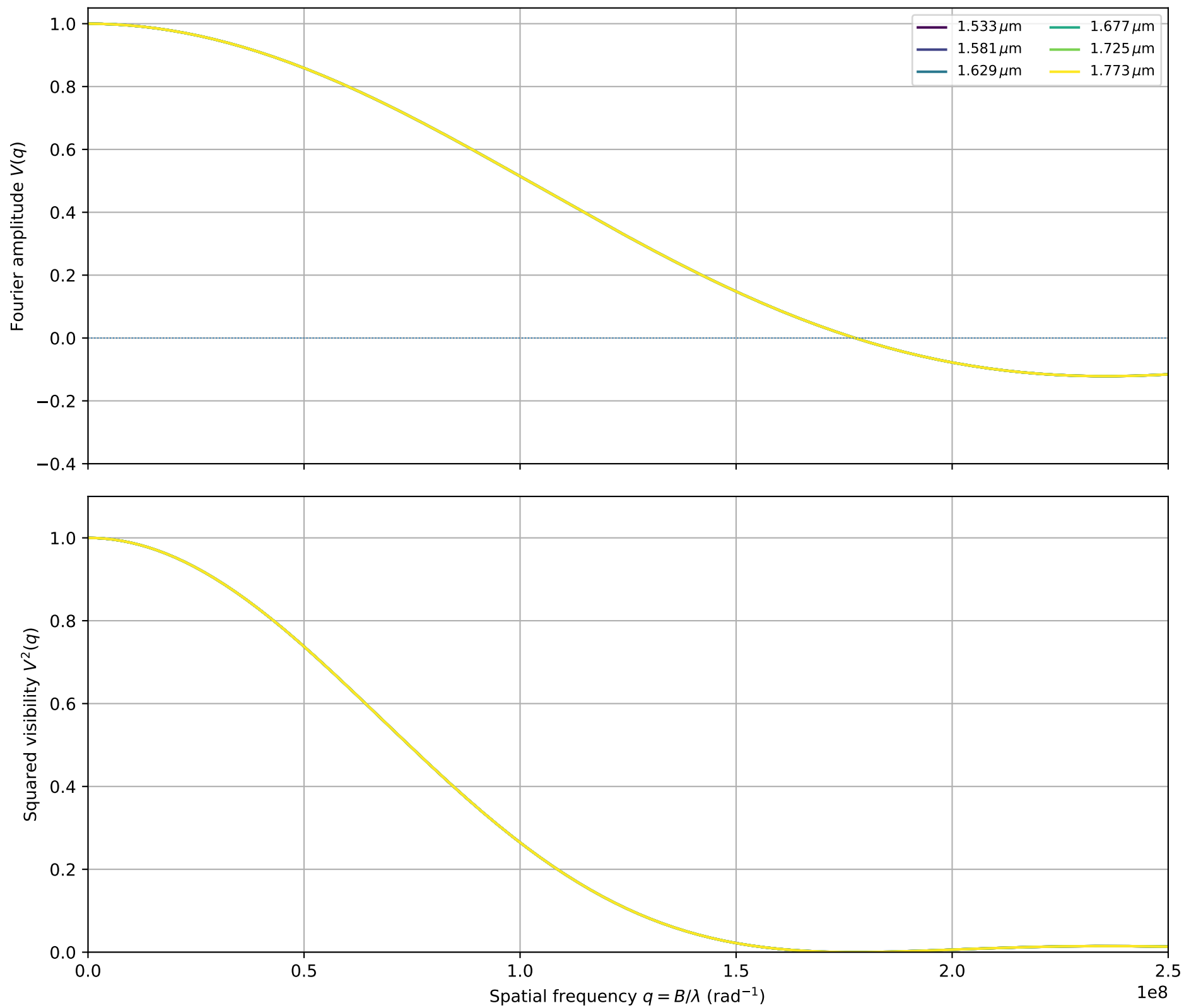
ksi_Gem: fitted \theta_{\text{LDD}} = 1.4555 \pm 0.0000 mas
