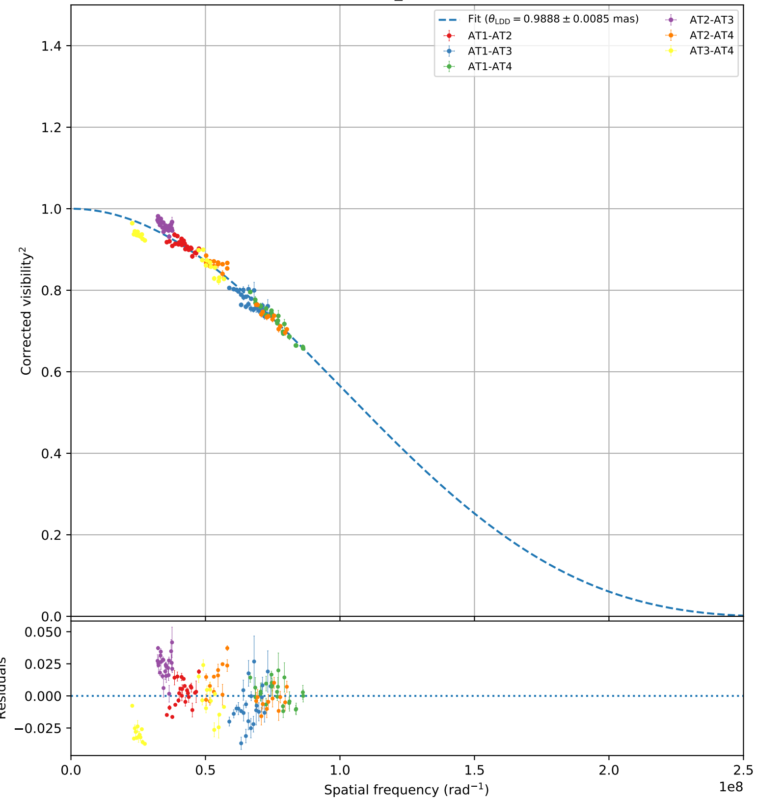
HR_2998
