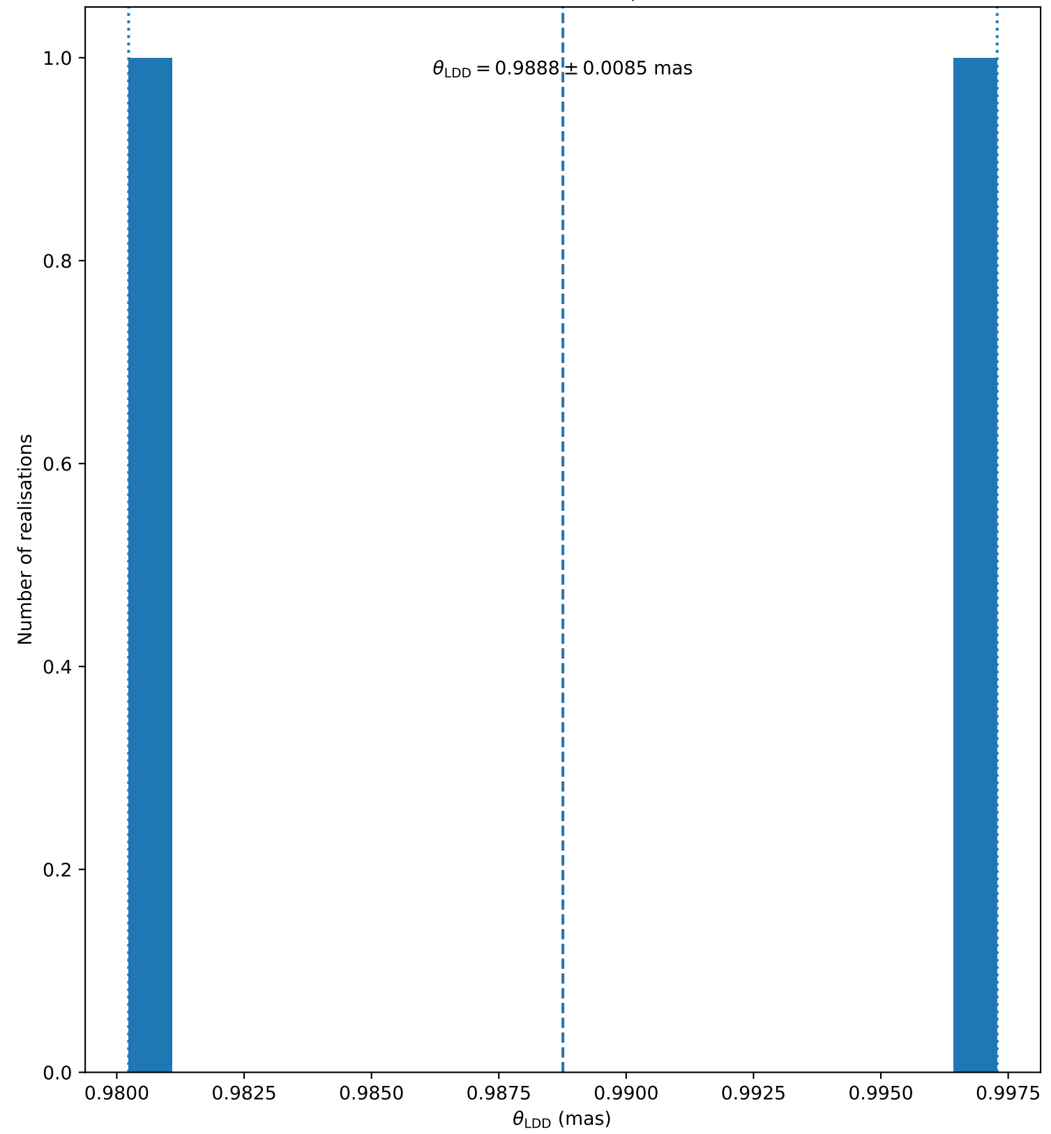
HR_2998 ( N_{\text{bootstrap}} = 2 )
