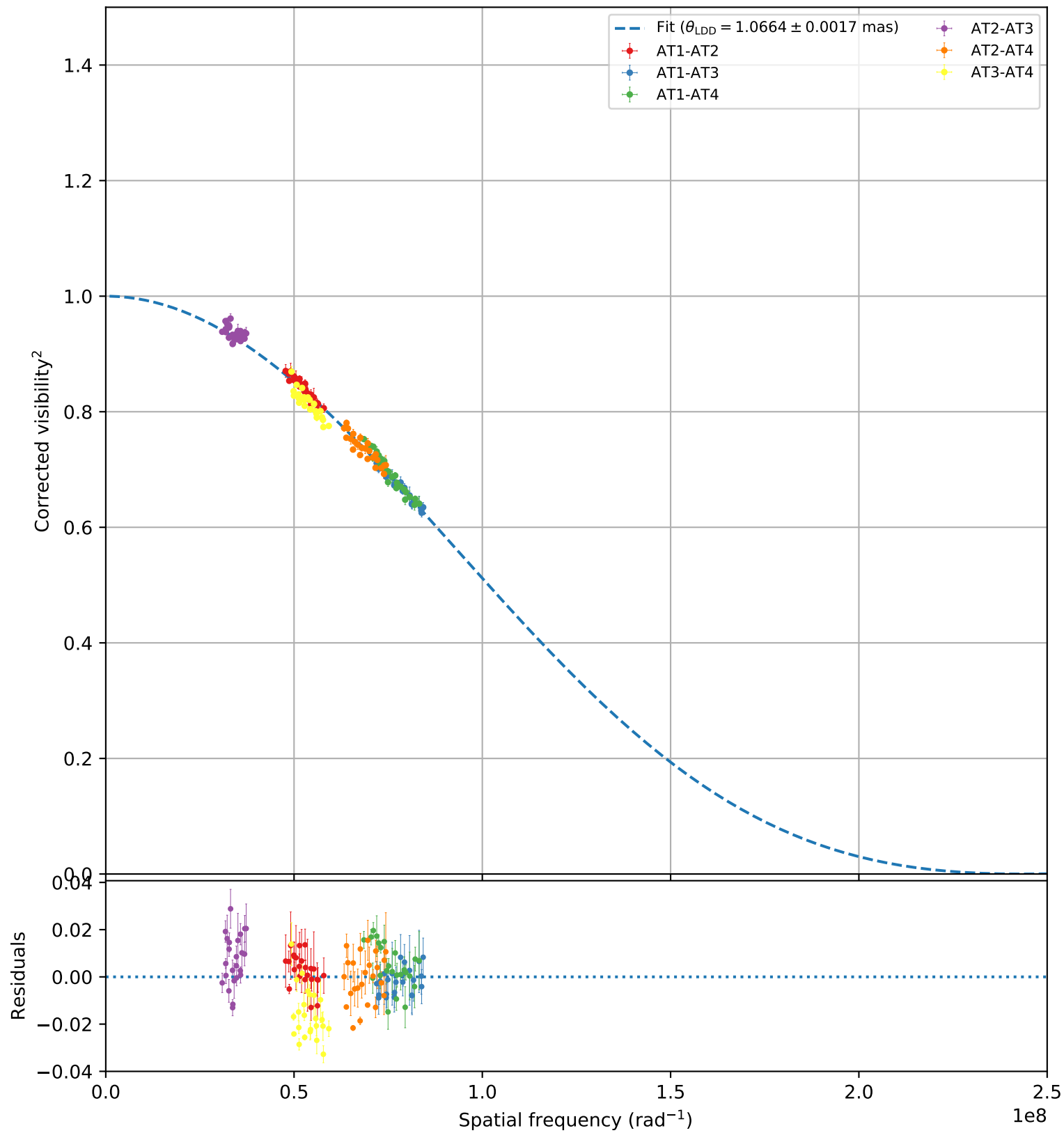
HD141004
