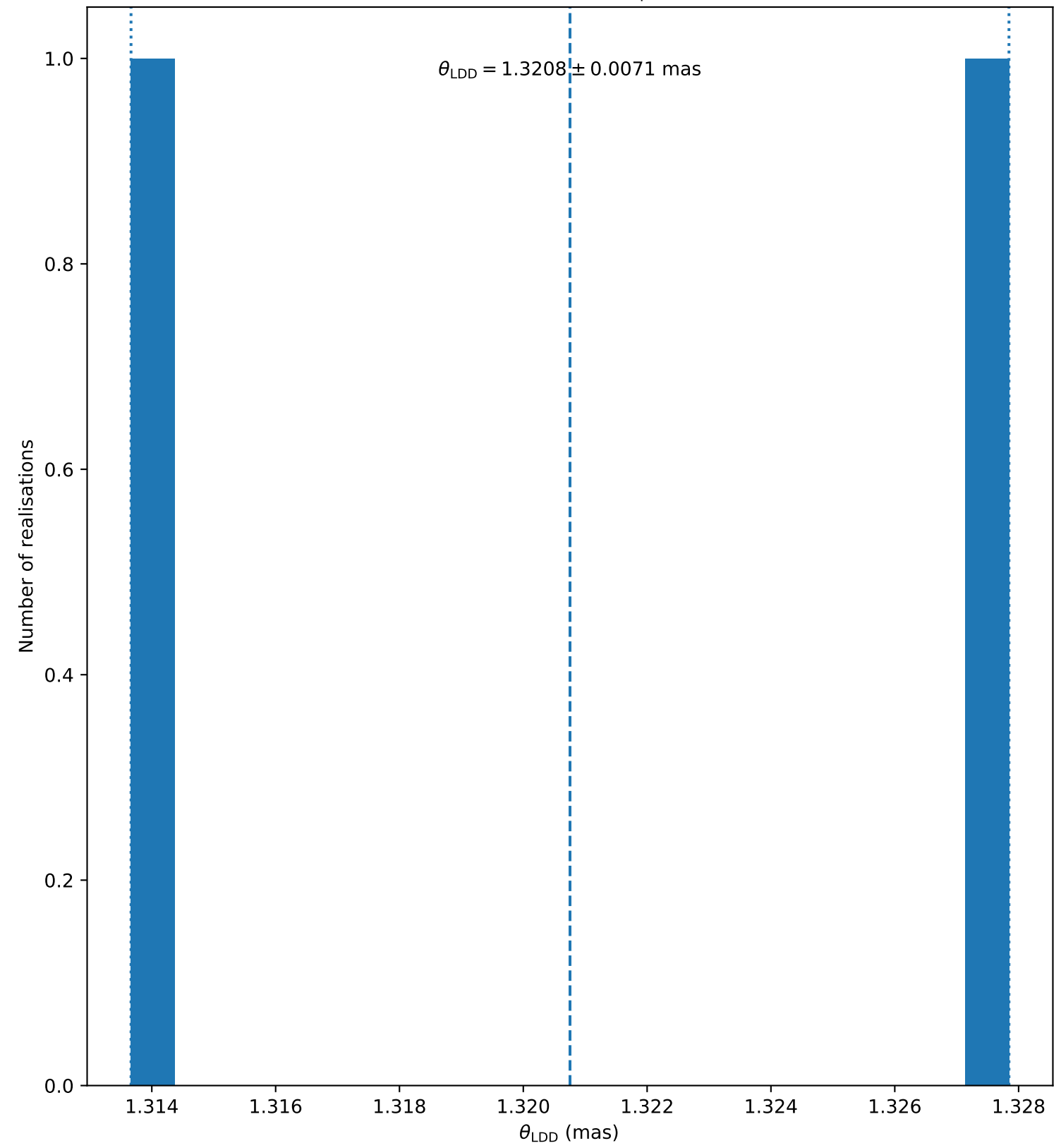
gam_Lep ( N_{\text{bootstrap}} = 2 )
