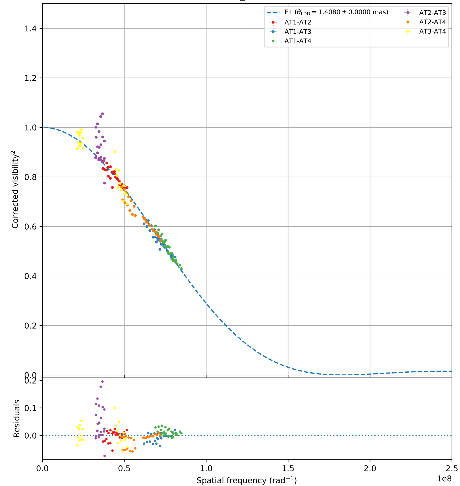
ksi_Gem
