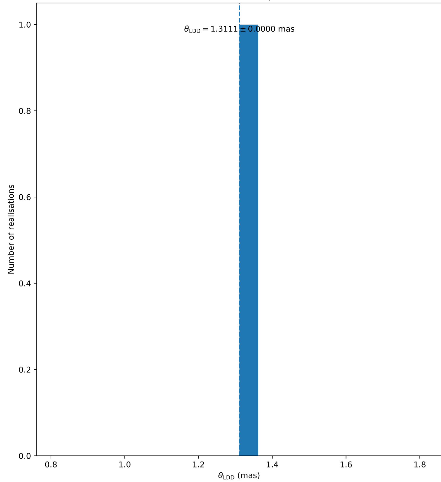
gam_Lep ( N_{\text{bootstrap}} = 1 )
