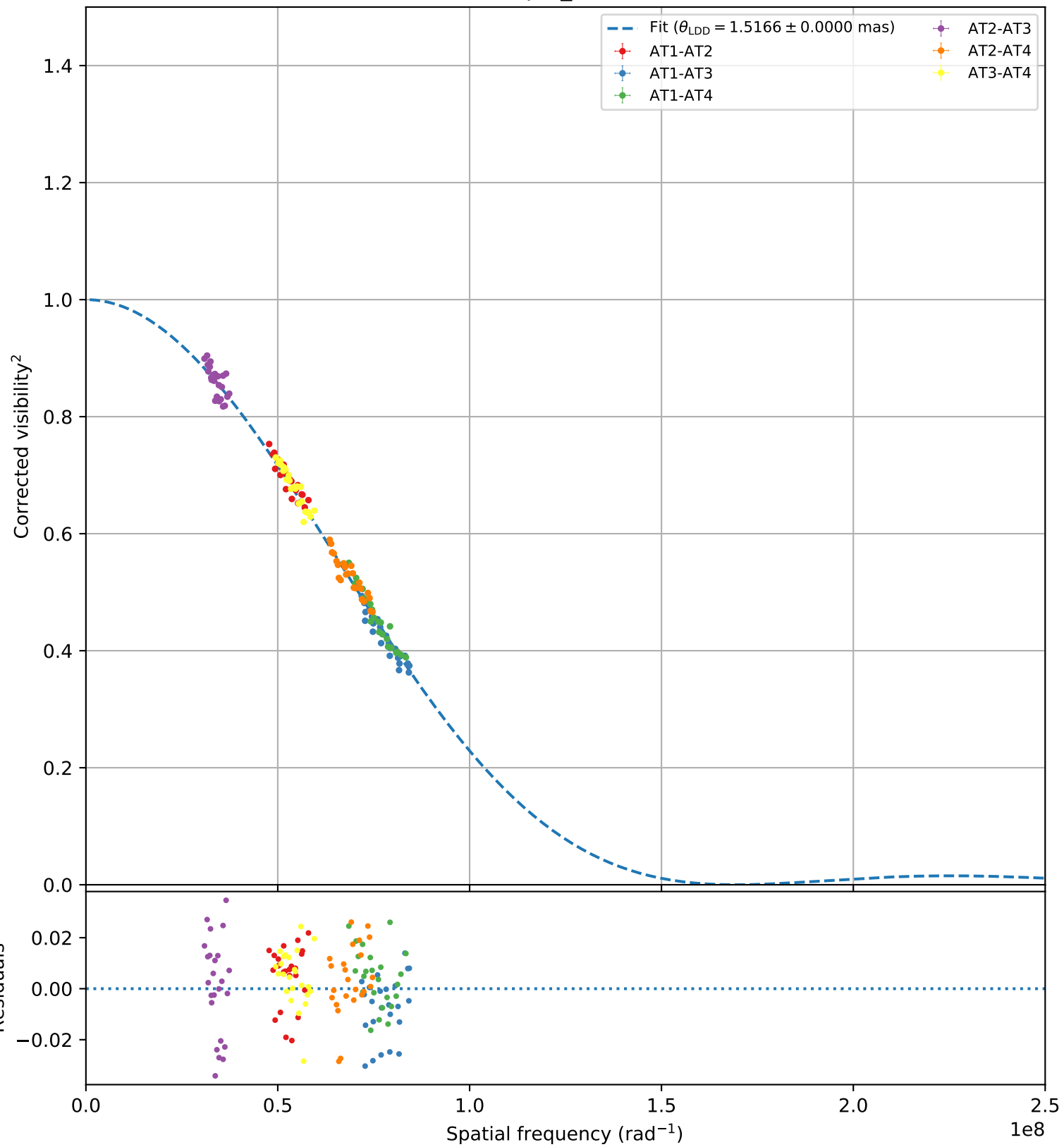
pi3_Ori
