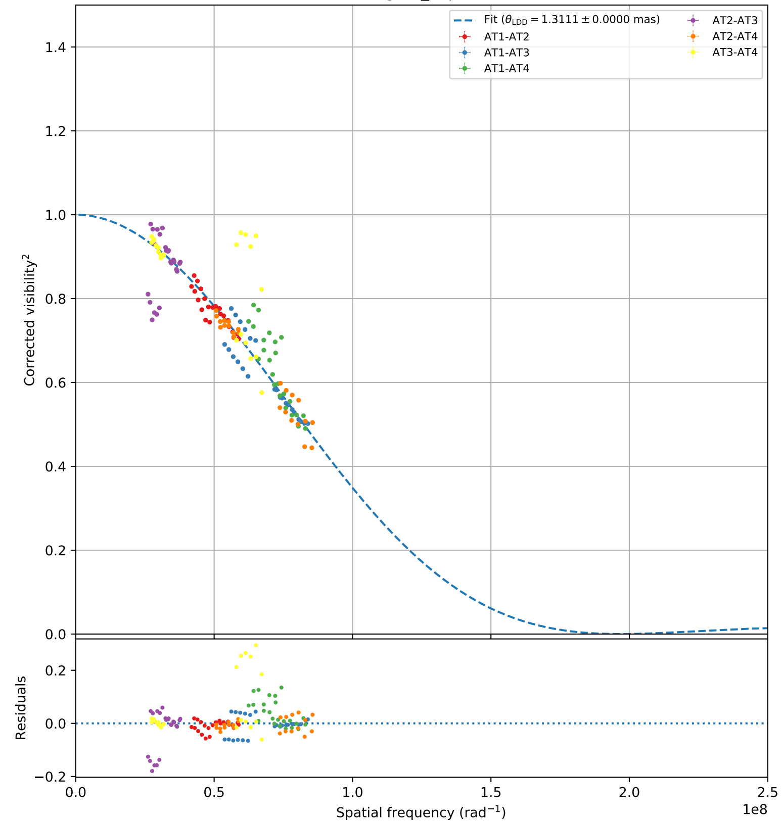
gam_Lep
