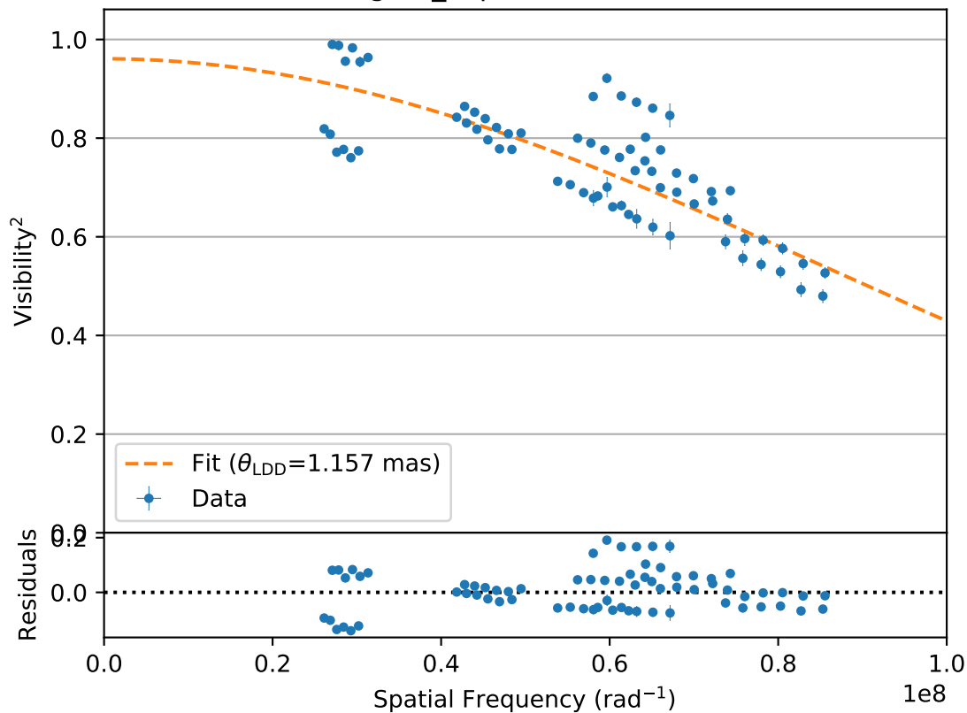
gam_Lep (faint, P106)
