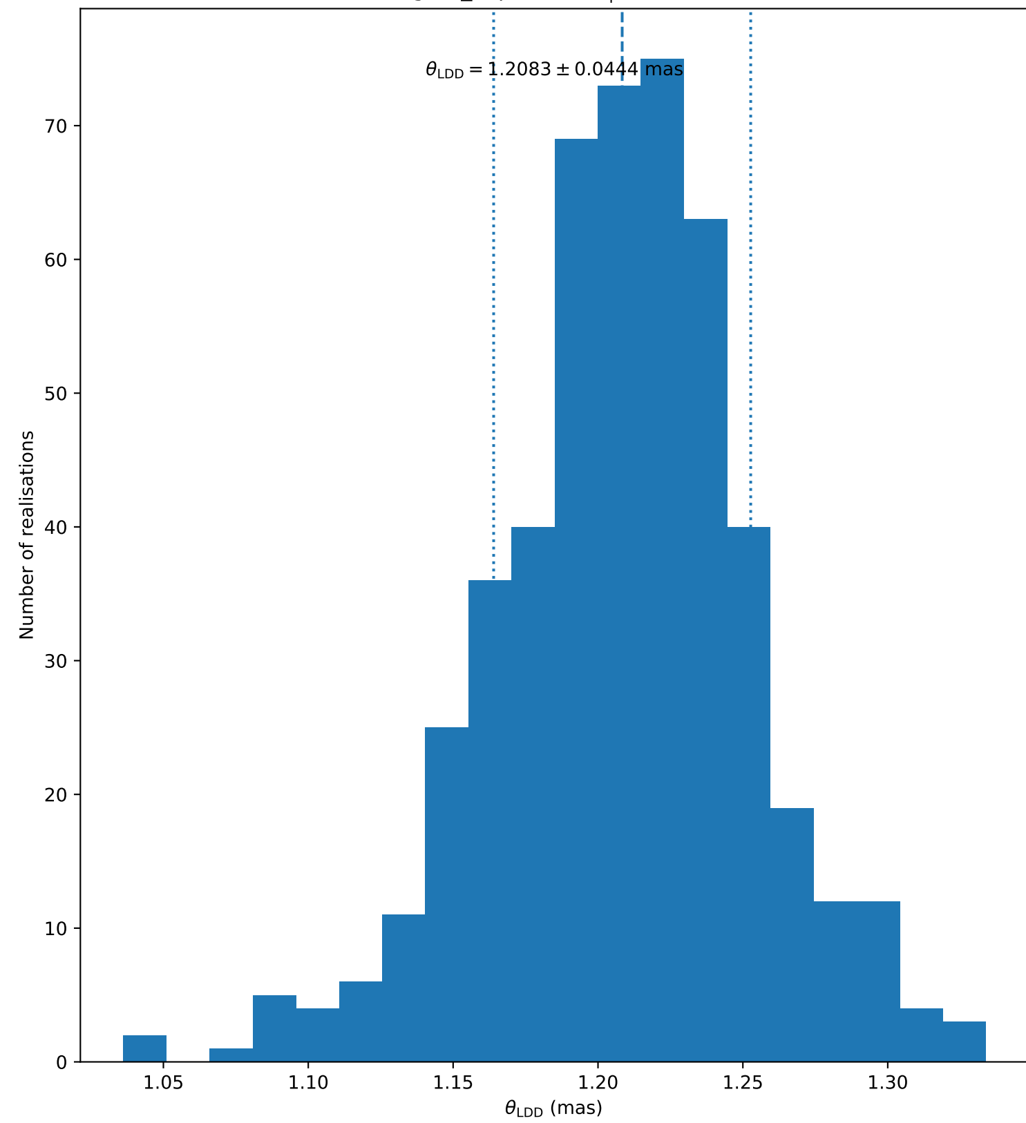
gam_Lep ( N_{\text{bootstrap}} = 500 )
