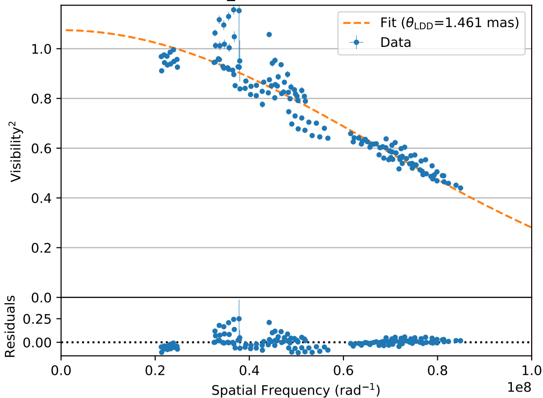
ksi_Gem (combined, P)
