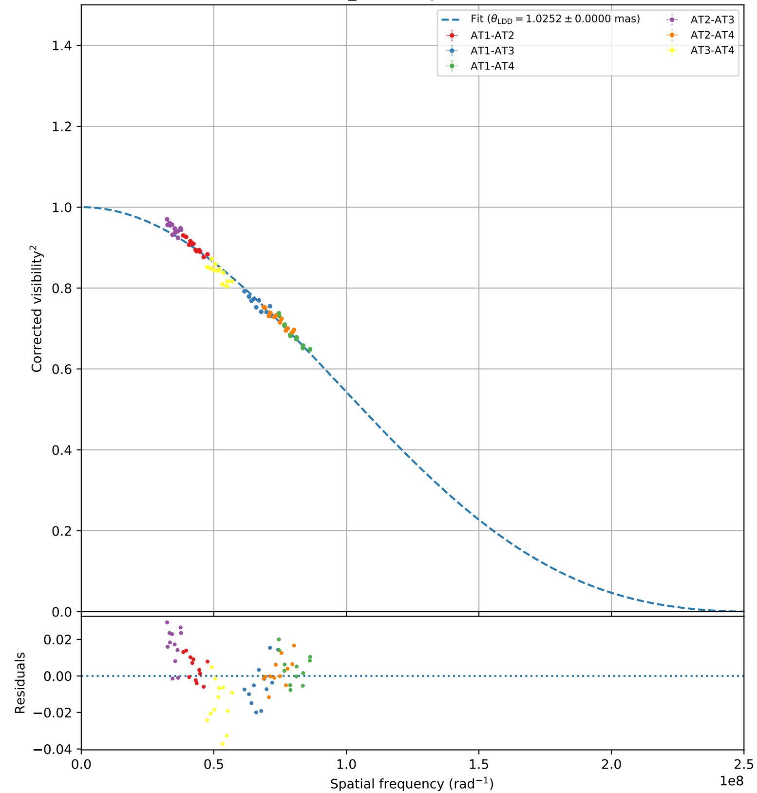
HR_2998 (bright, 104)
