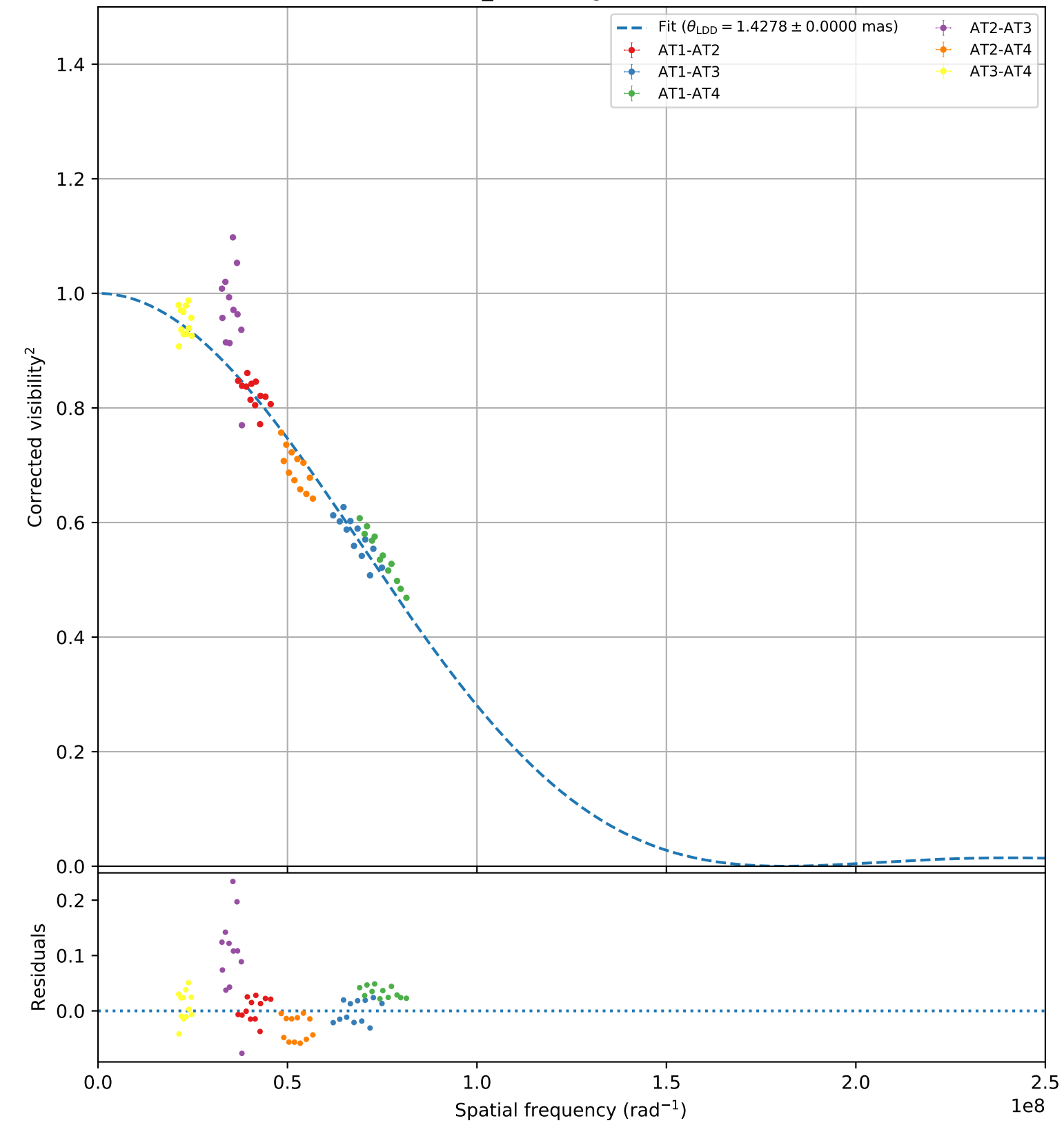
ksi_Gem (bright, 106)
