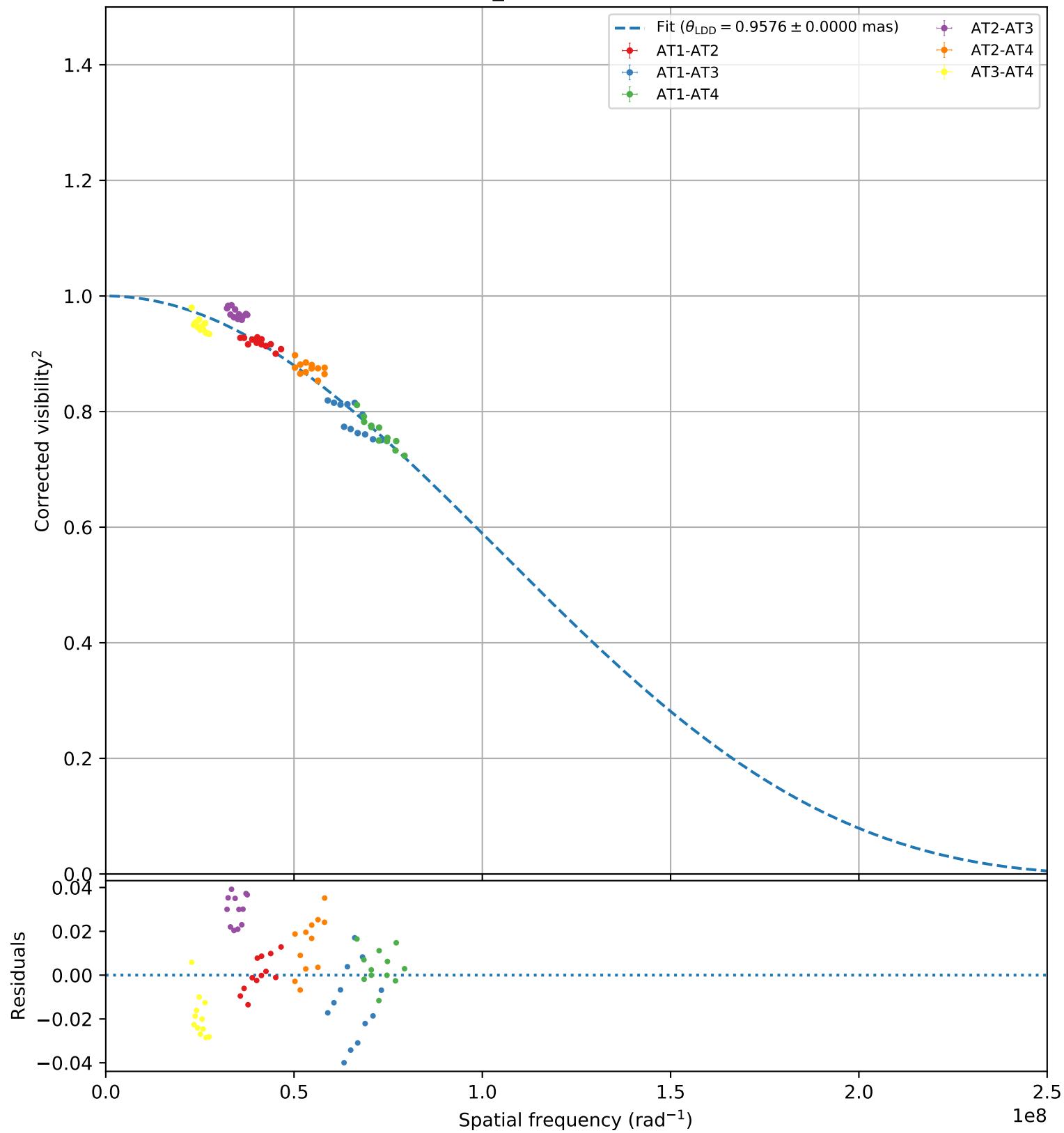
HR_2998 (faint, 104)
