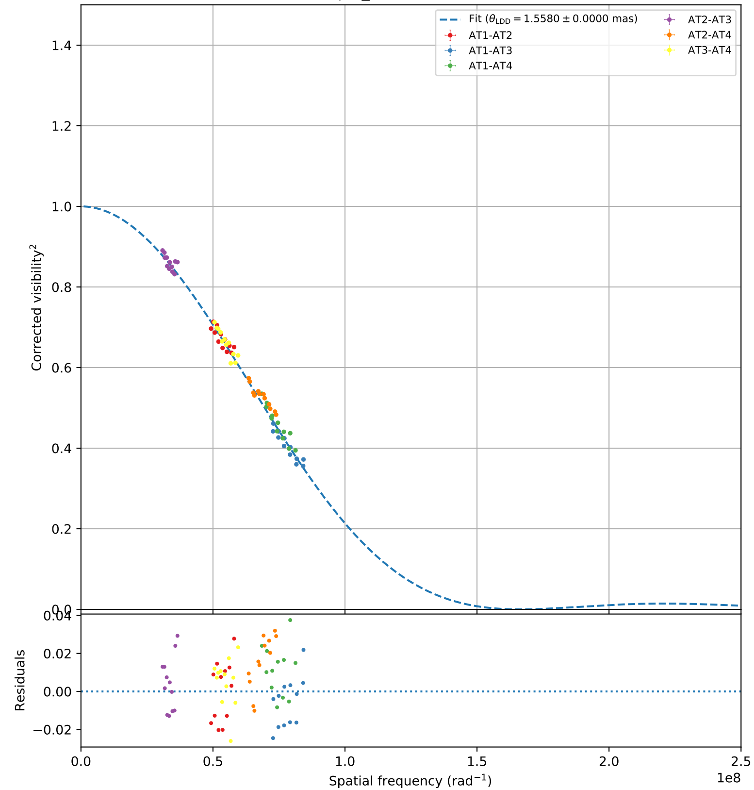
pi3_Ori (faint, 104)
