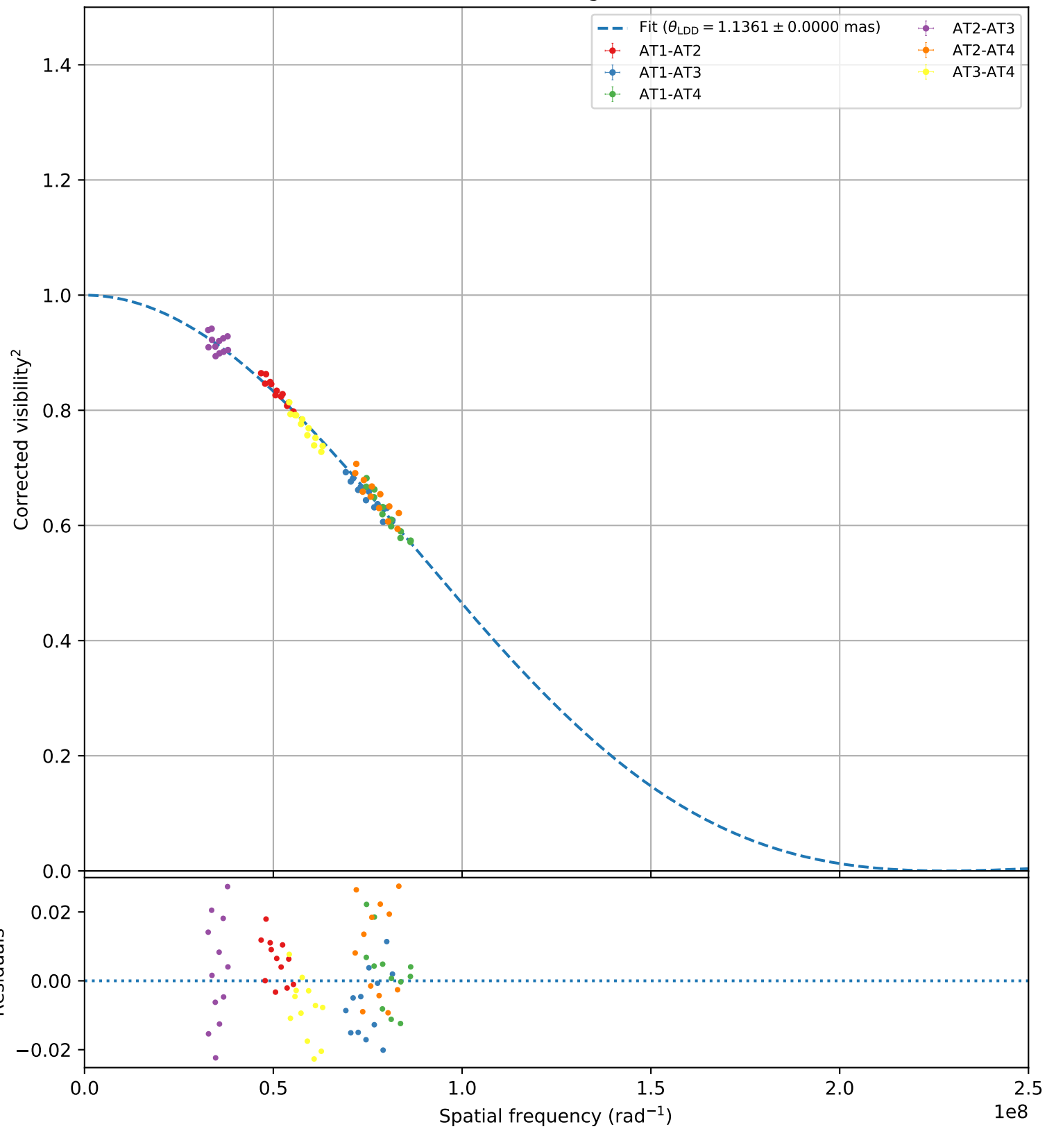
HD124850 (bright, 105)
