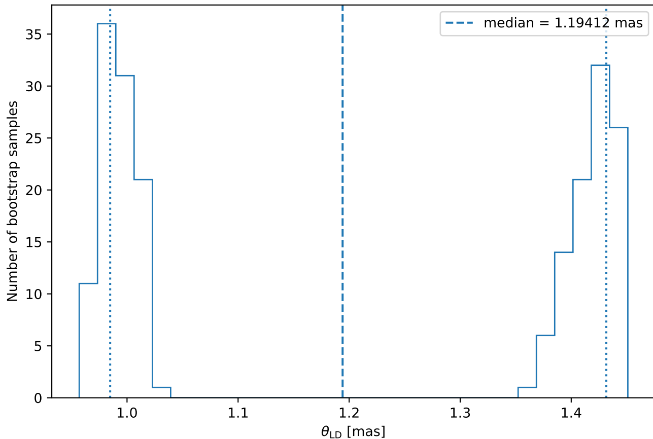
ksi Gem - ALL
