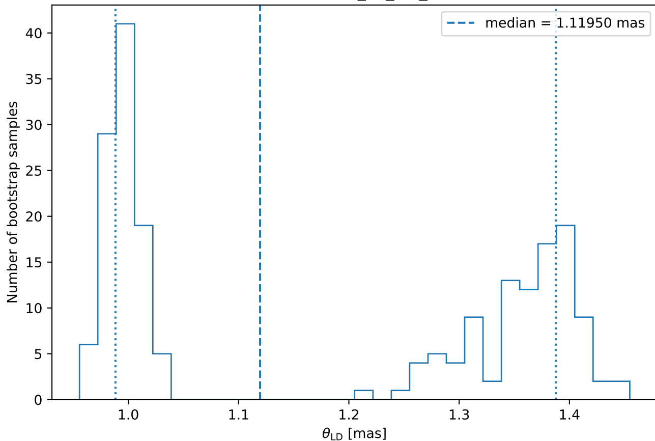
ksi Gem - NO_BL_NO_CAL
