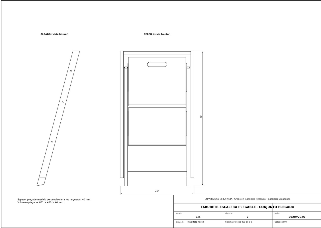
Plano 2. Conjunto plegado.
