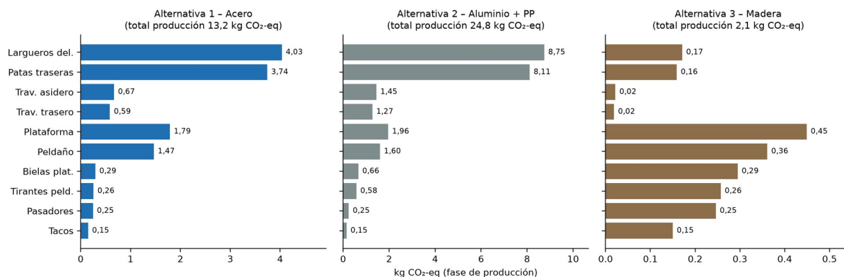
Ilustración 18. Huella de carbono de la fase de producción por componente. Elaboración propia.
