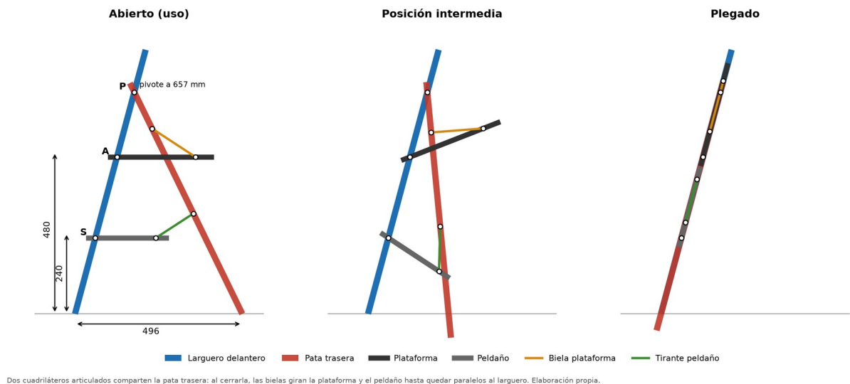
Ilustración 13. Esquema cinemático definitivo: posiciones abierta, intermedia y plegada. Elaboración propia.
