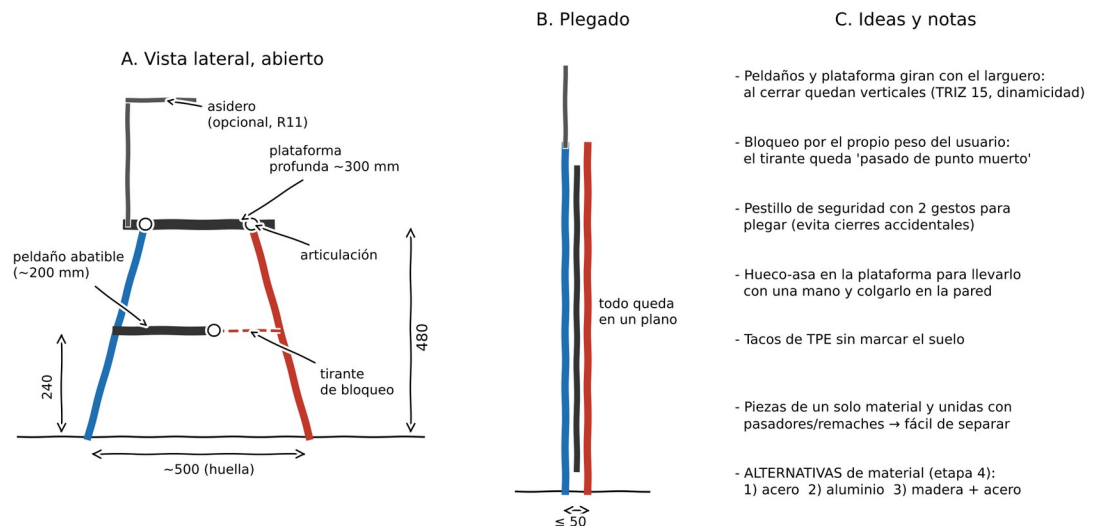
Ilustración 12. Boceto inicial del concepto. Elaboración propia.
