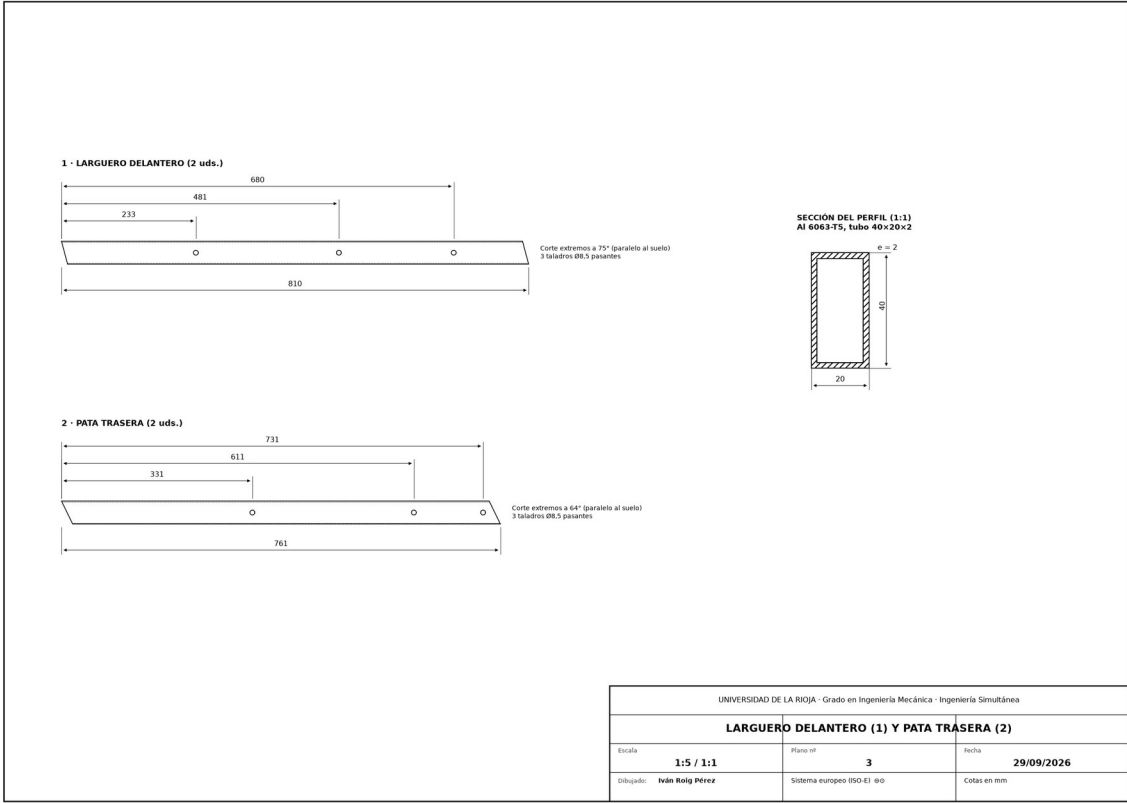
Plano 3. Larguero delantero y pata trasera.
