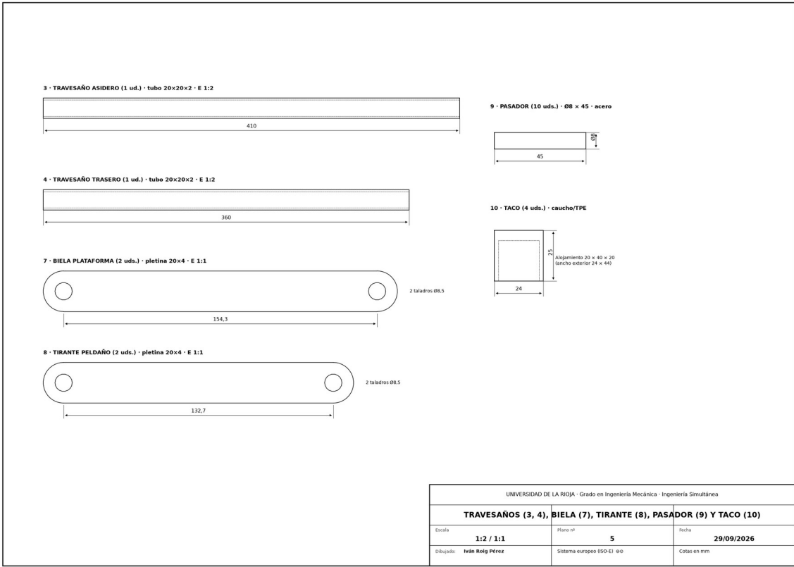
Plano 5. Travesaños, biela, tirante, pasador y taco.
