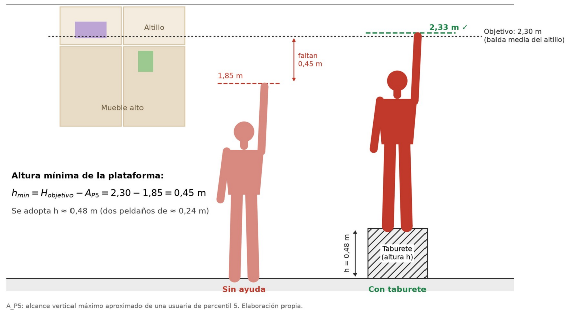
Ilustración 3. Determinación de la altura de la plataforma superior. Elaboración propia.
