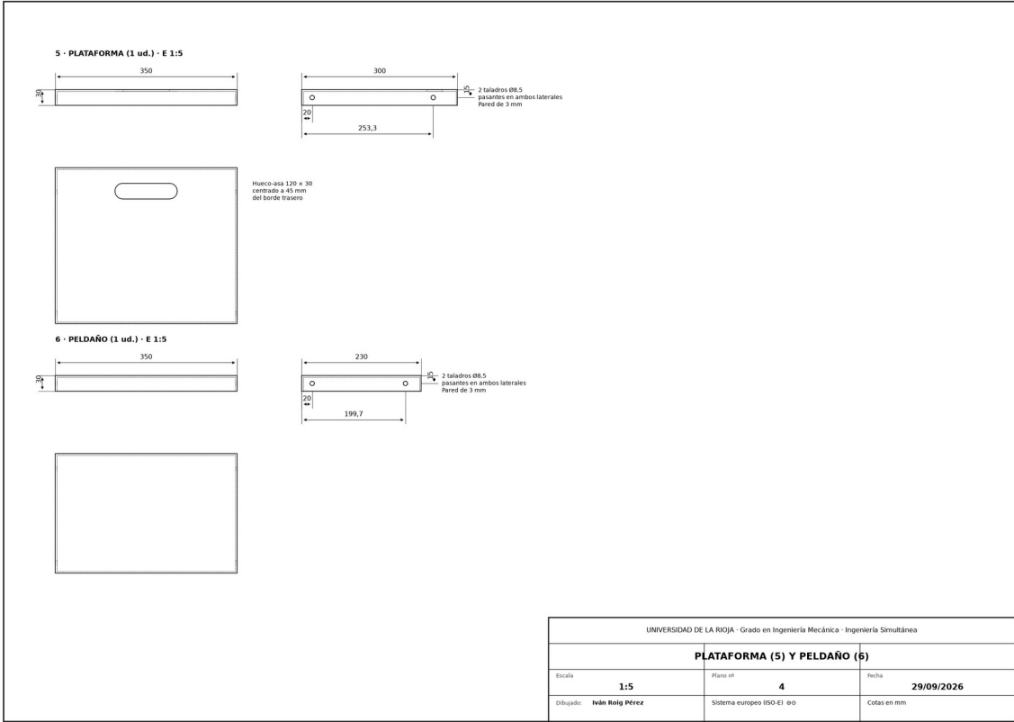
Plano 4. Plataforma y peldaño.
