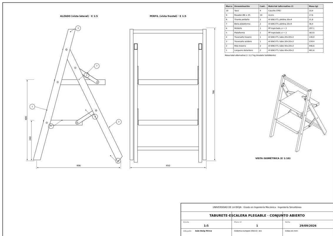
Plano 1. Conjunto abierto con lista de piezas.
