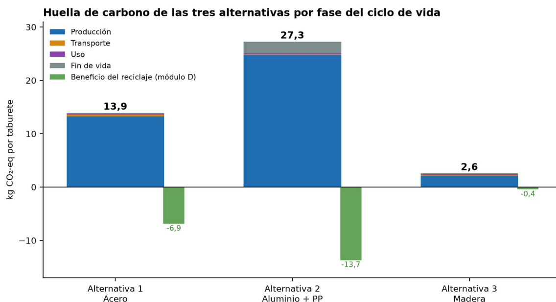
Ilustración 17. Huella de carbono de las tres alternativas por fase del ciclo de vida. Elaboración propia.
