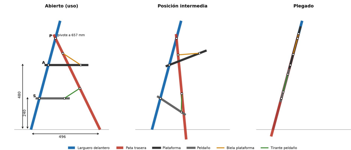
Esquema cinemático definitivo del mecanismo de plegado (cotas en mm)
