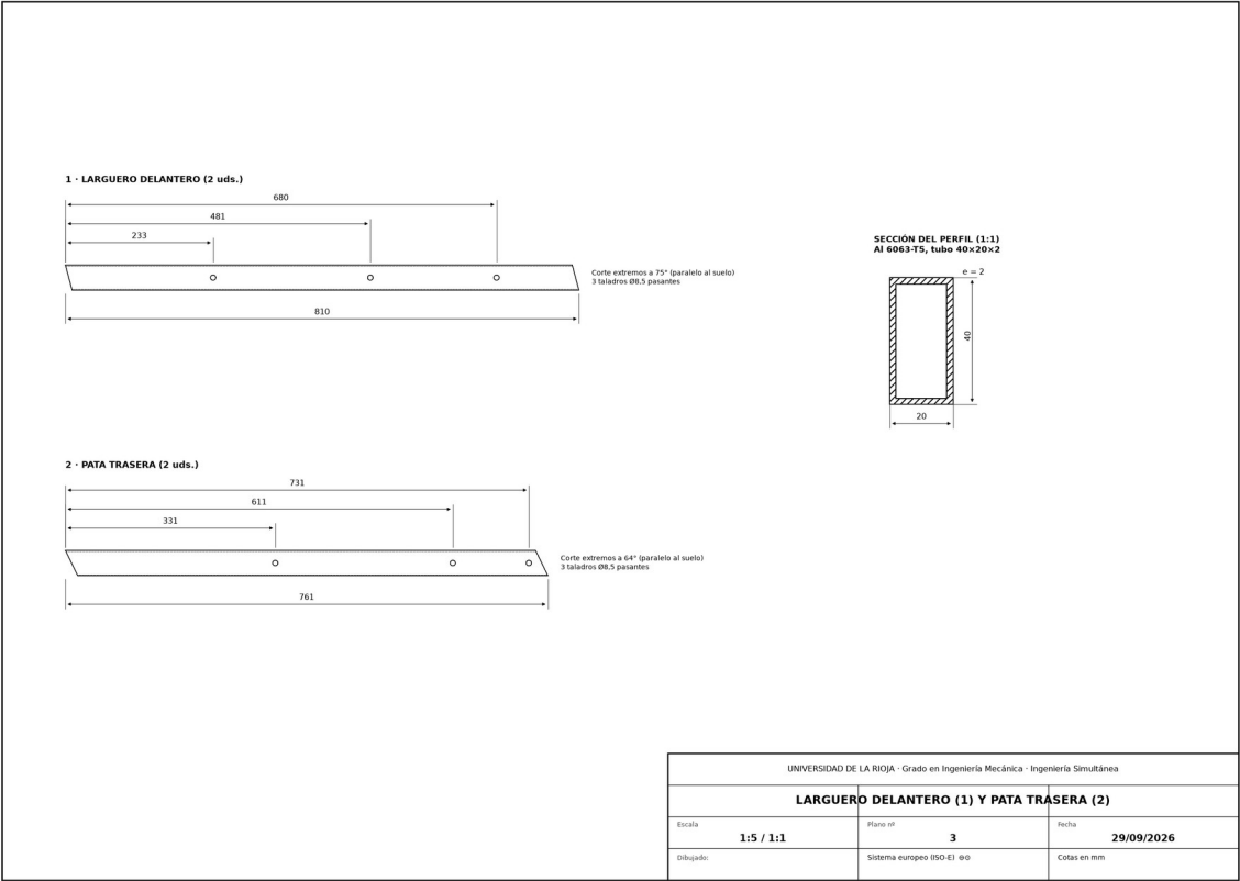
Plano 3. Larguero delantero y pata trasera.
