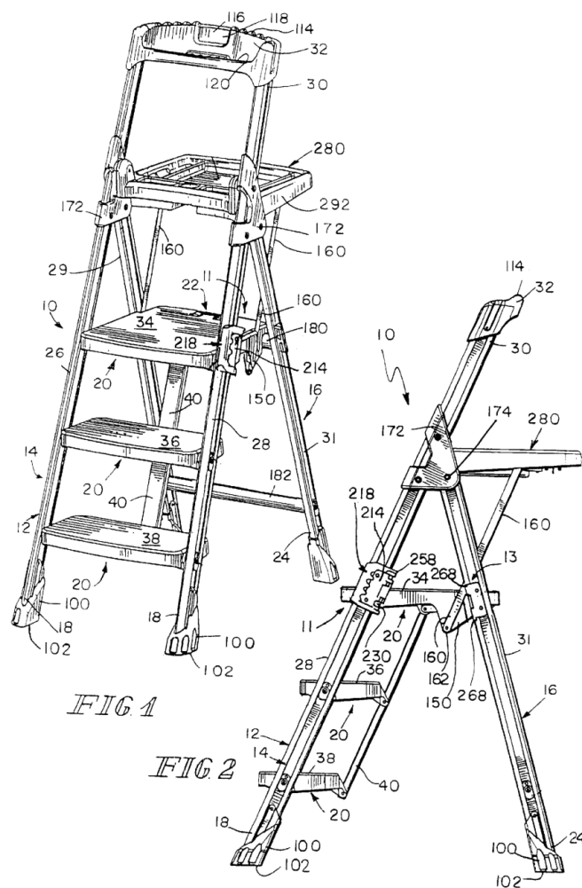
Ilustración 7. Figuras 1 y 2 de la patente US 6 454 050 B2. Fuente: USPTO / Google Patents.
