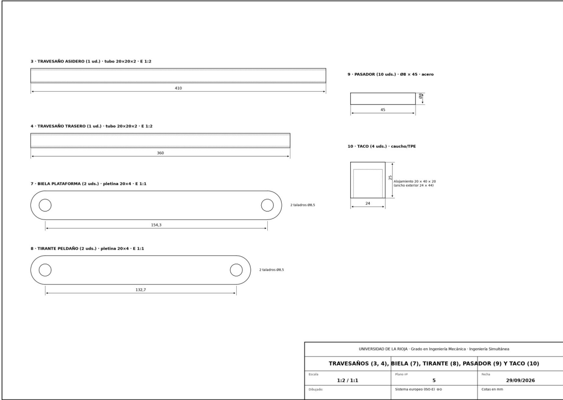
Plano 5. Travesaños, biela, tirante, pasador y taco.
