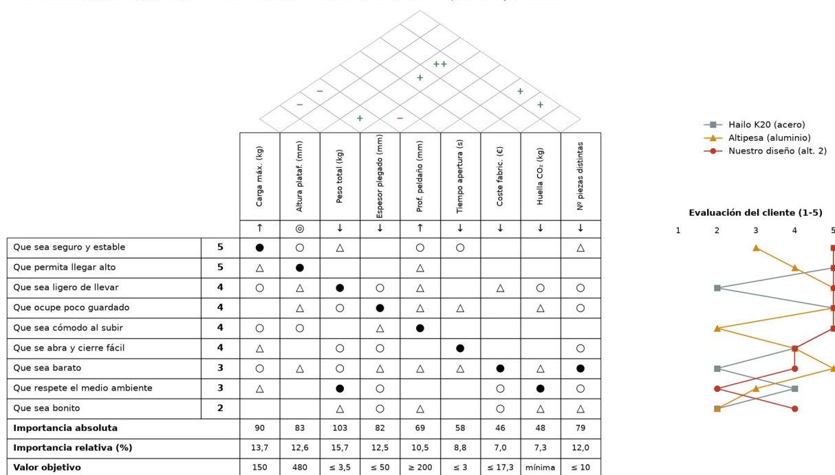
Casa de la calidad (QFD) del taburete-escalera
