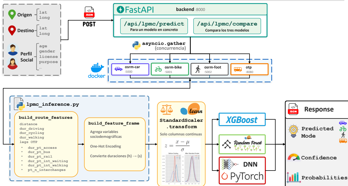
Figura 4.3: Pipeline de inferencia de elección modal.
