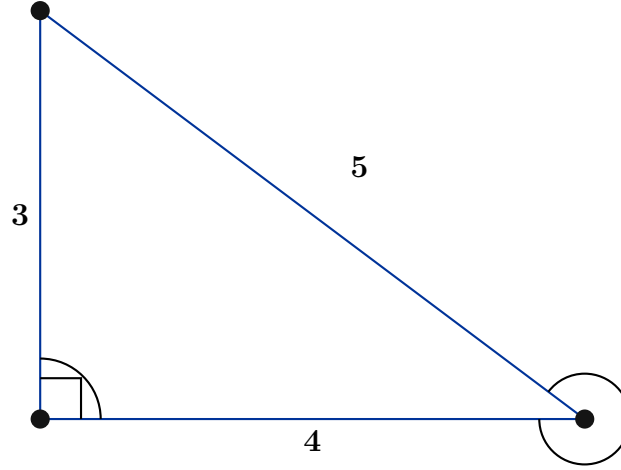
Figura 1: El Triángulo Sagrado 3-4-5 y sus ángulos fundamentales.
