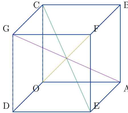
Figura 3: El cubo de Russell con sus 3 diagonales espaciales (planos de simetría).
