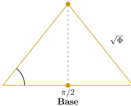
Figura 2: Sección transversal de la Gran Pirámide mostrando el ángulo de inclinación 51,84°.
