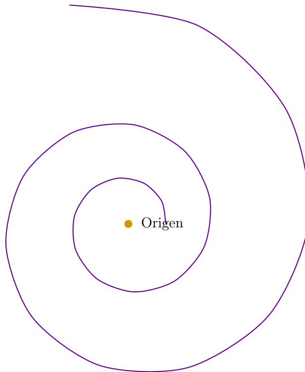
Figura 5: La espiral logarítmica áurea: el patrón fundamental del vórtice cósmico.
