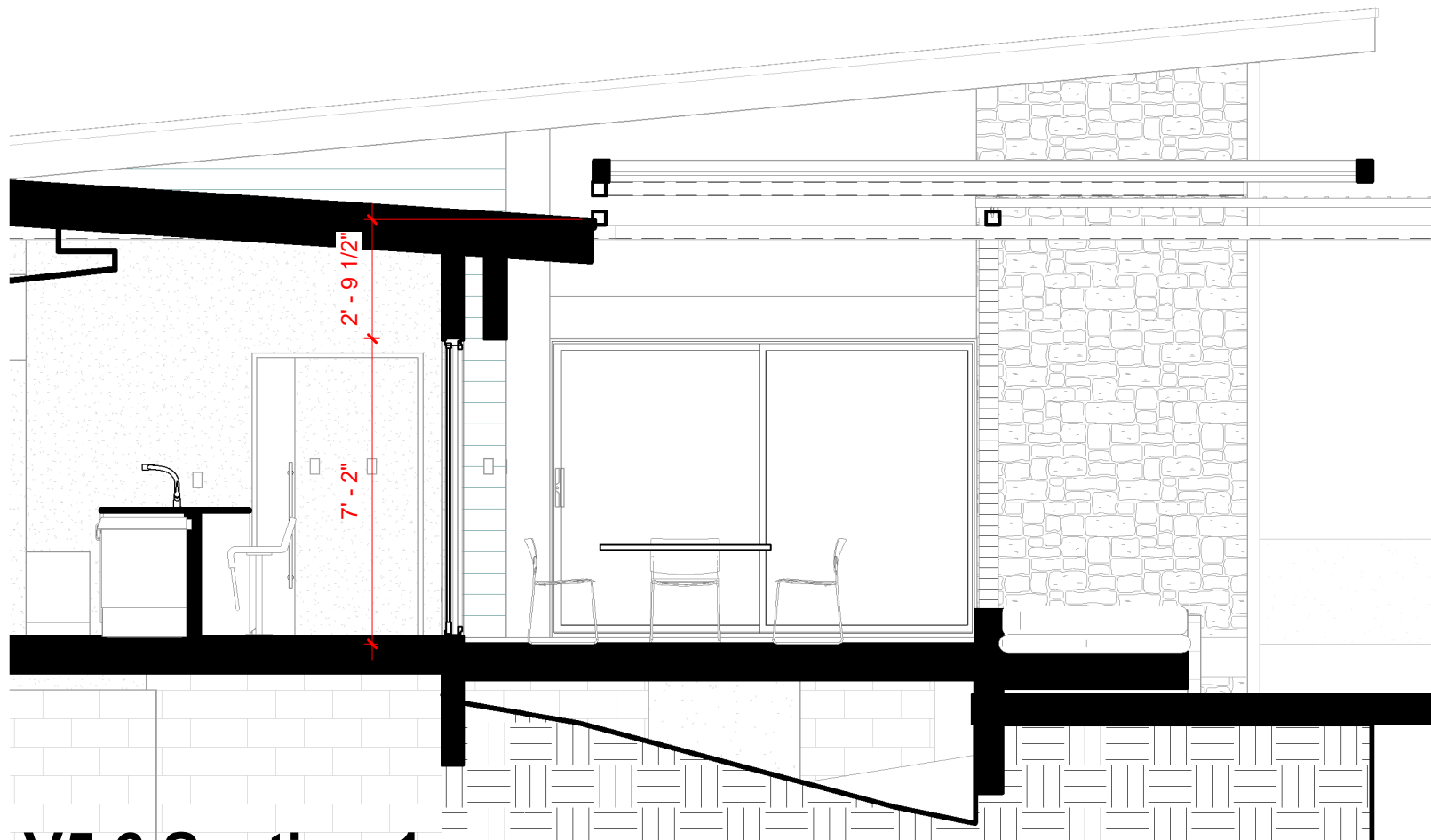
V5.6.Section.1 1/4" = 1'-0"
