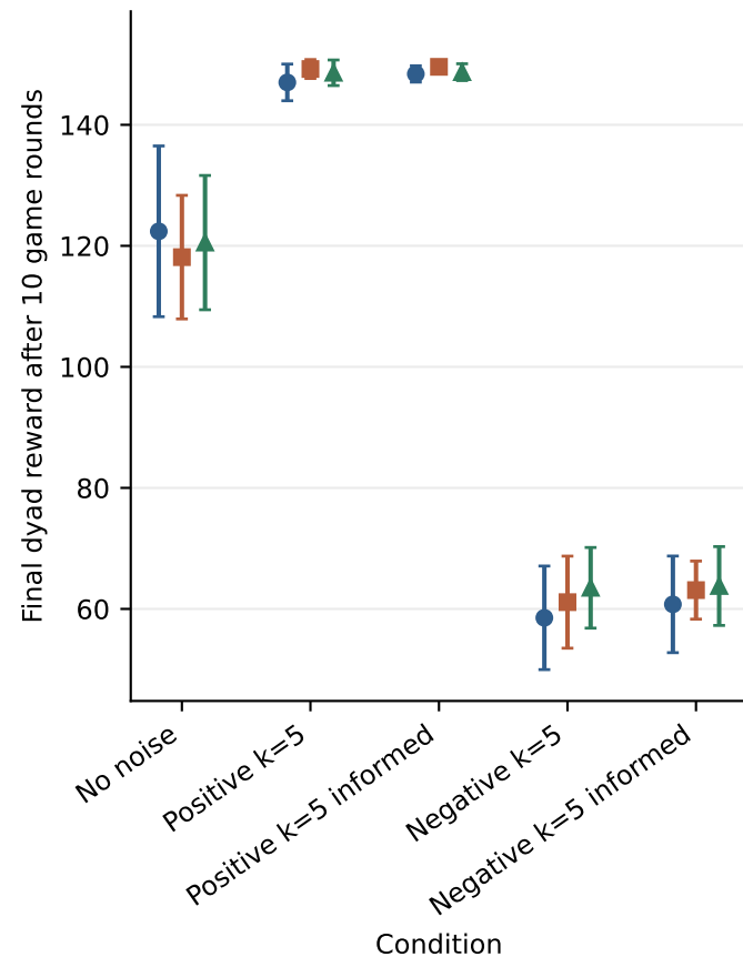
Claude Sonnet 4.5
